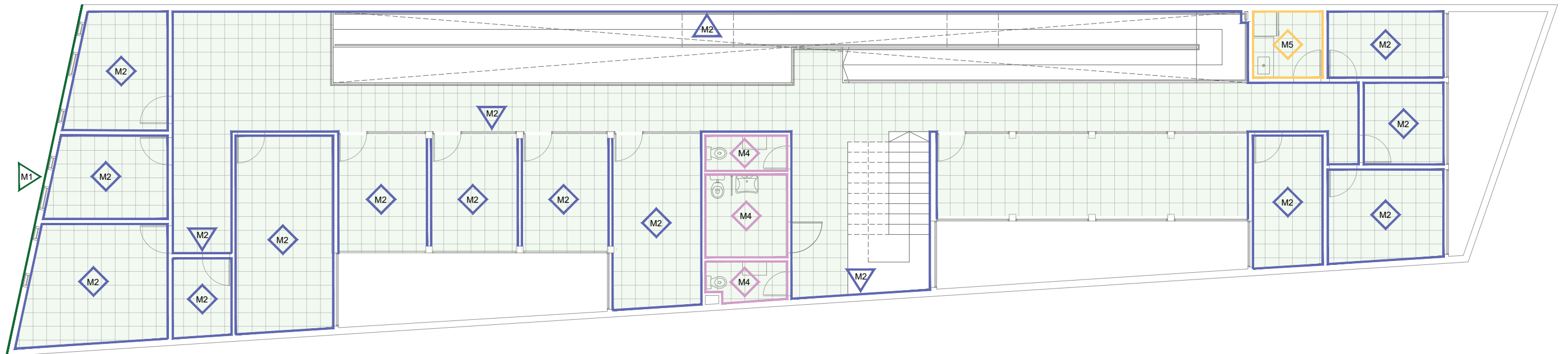
PLANTA ALTA
