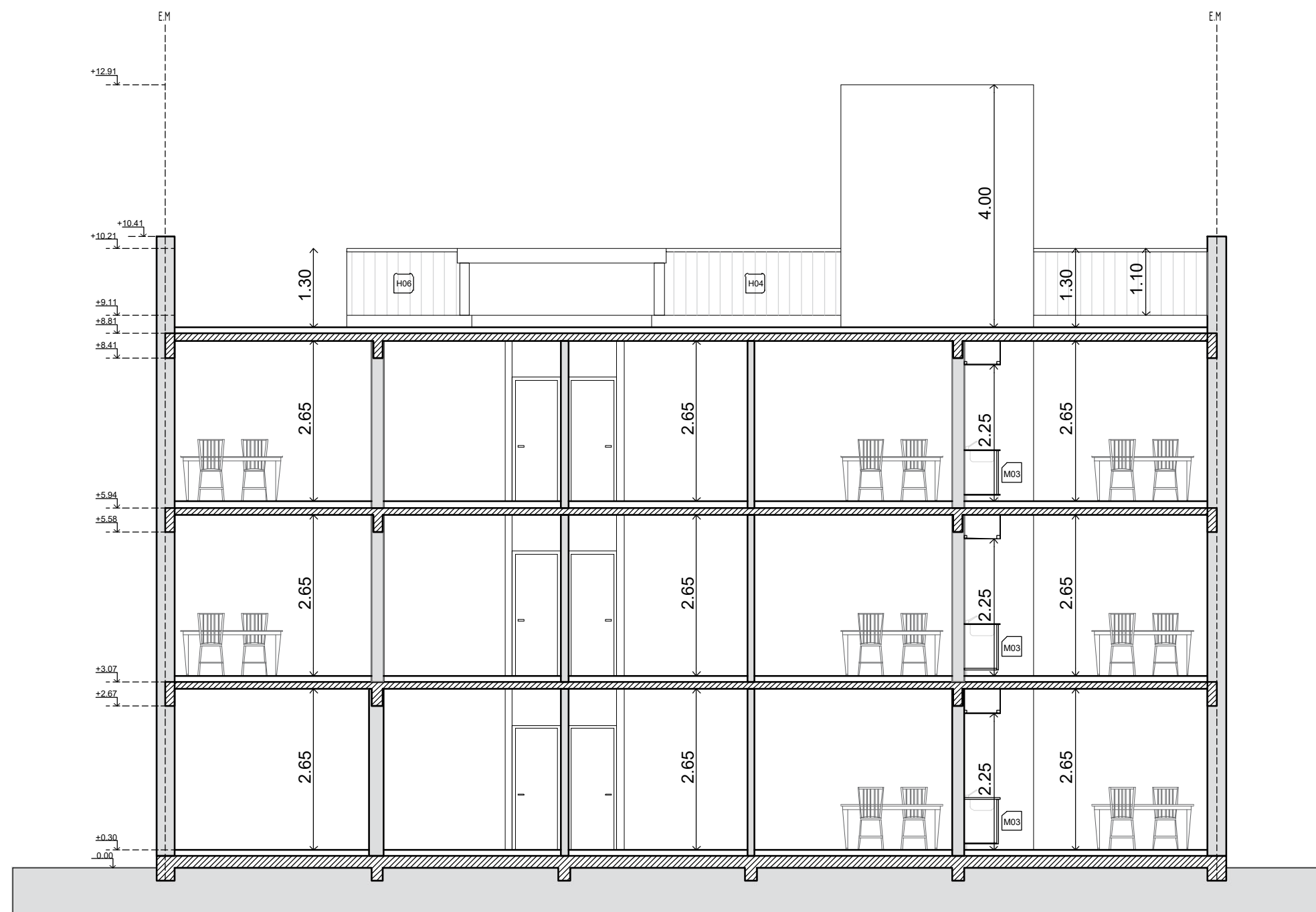
CORTE A.A
