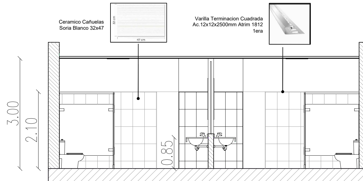
CORTE A-A
