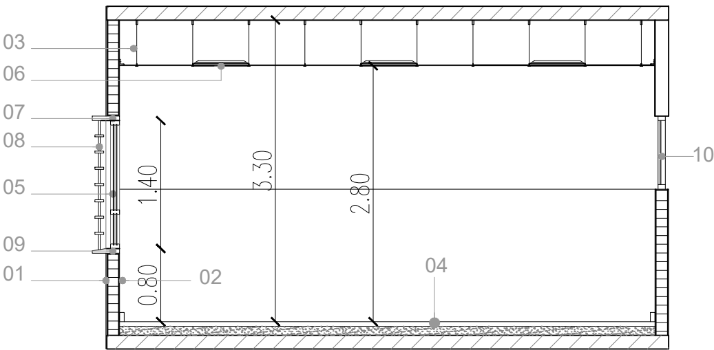
CORTE AULA
