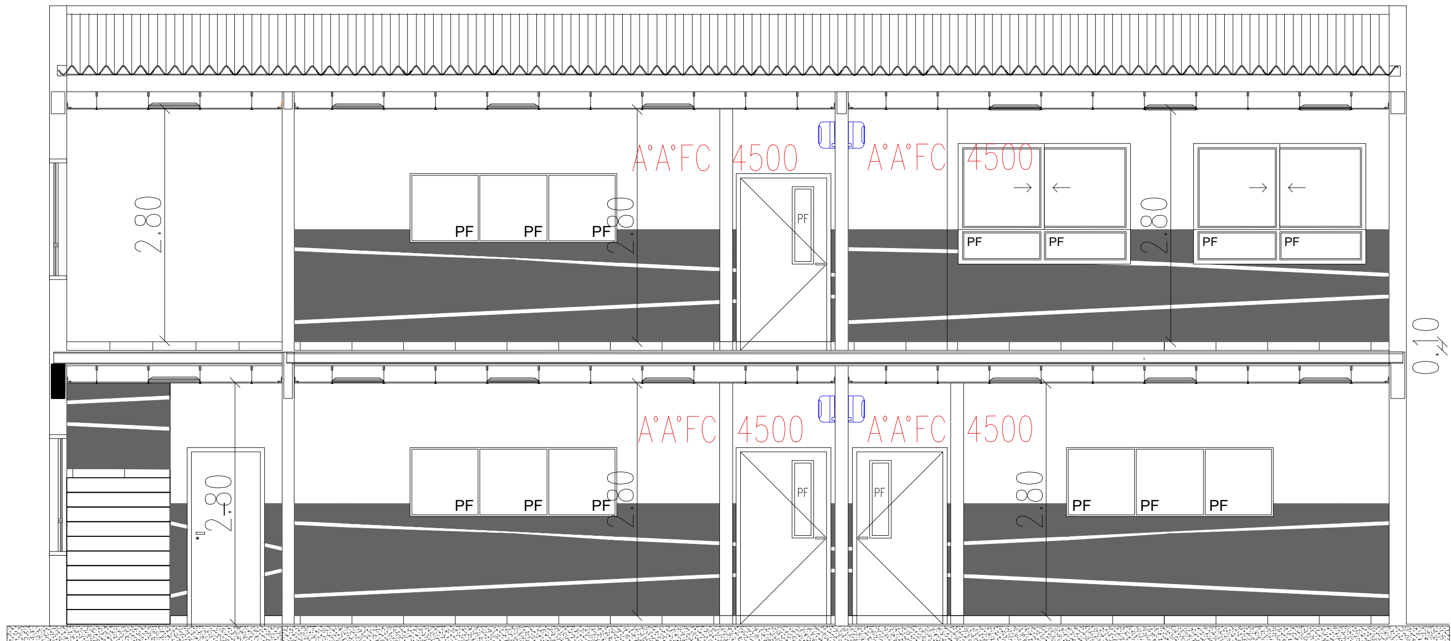
CORTE A-A
