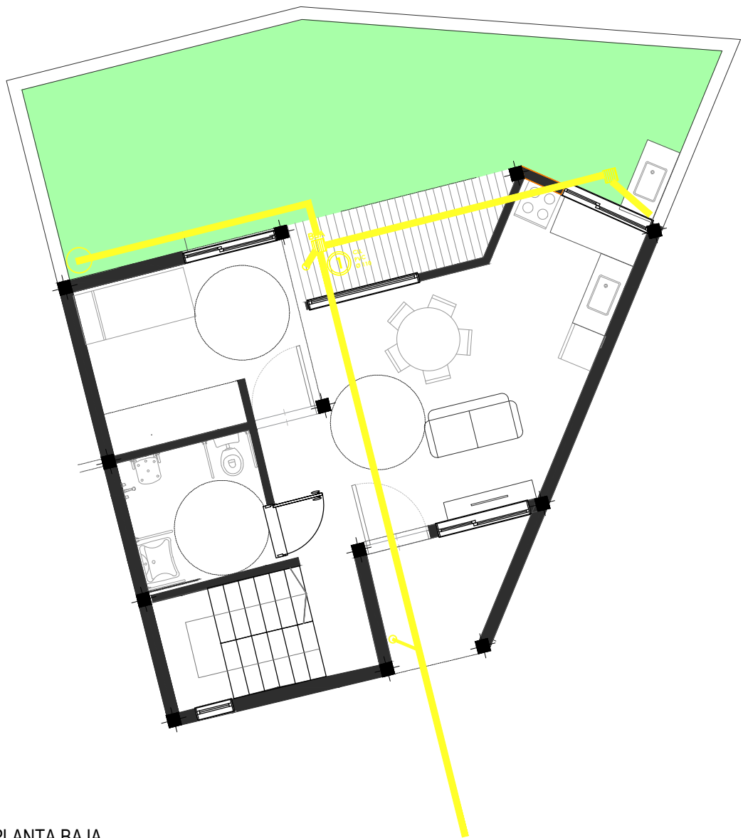
PLANTA BAJA
