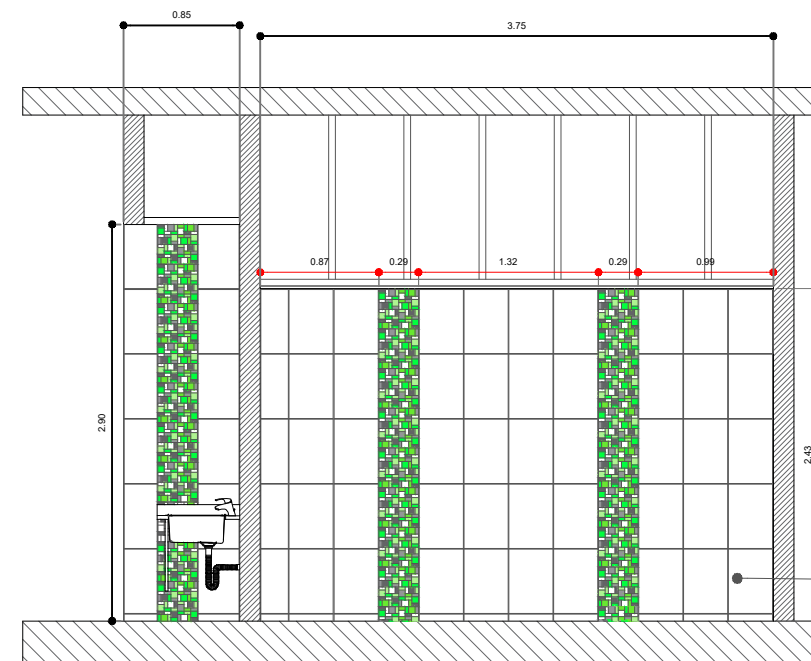
CORTE B-B
