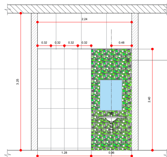
CORTE B-B
