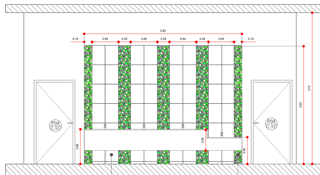
VISTA A
