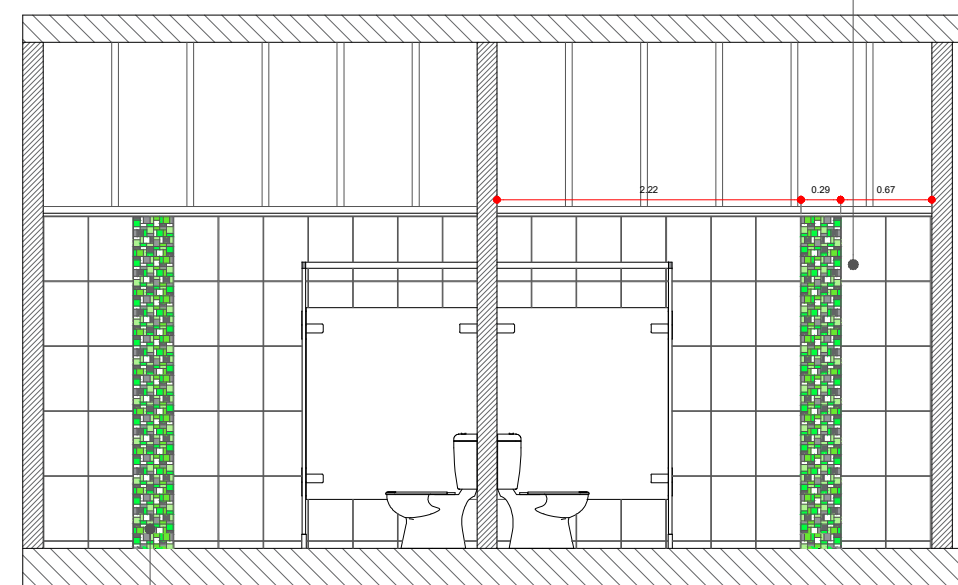
CORTE C-C
