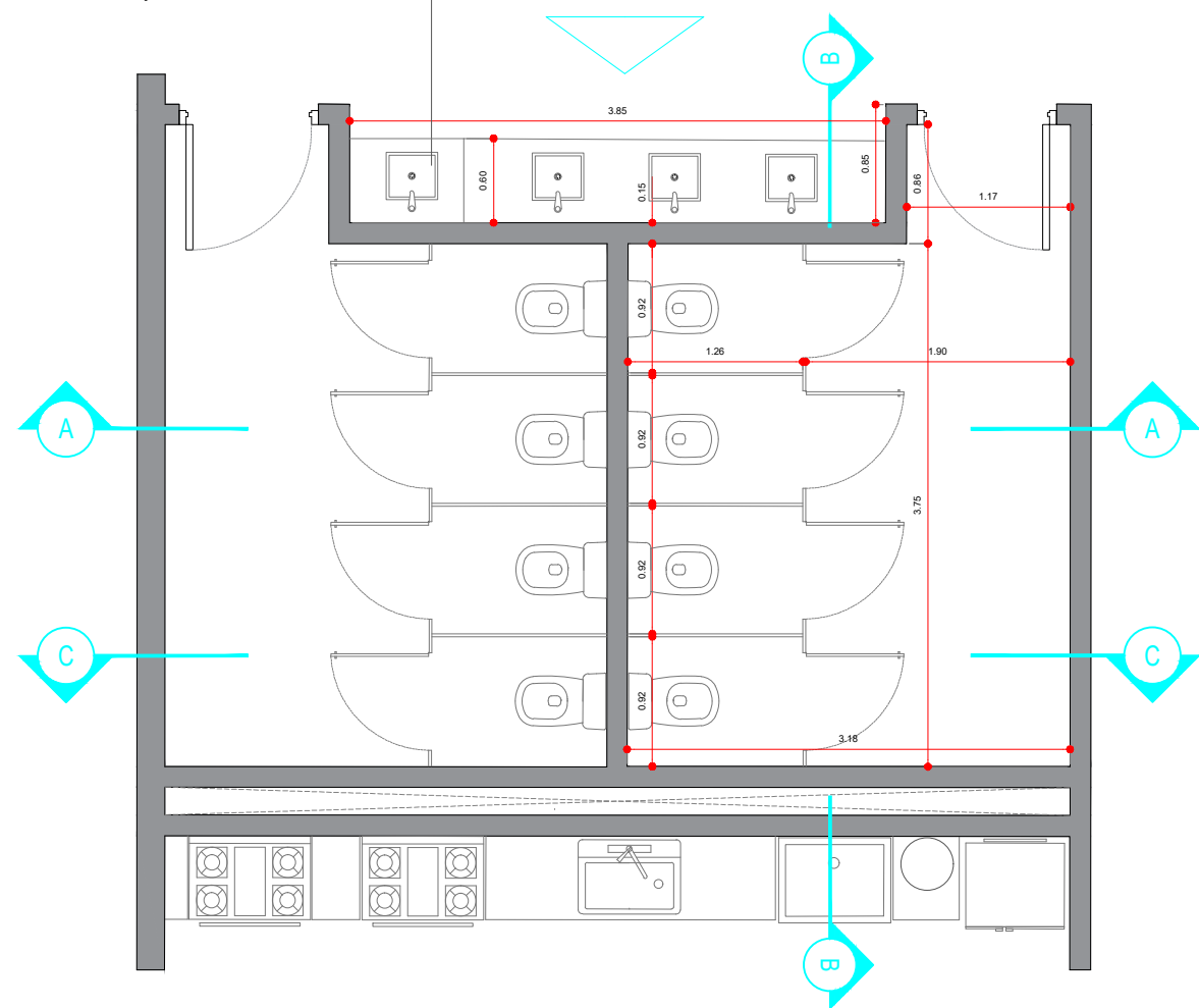
VISTA A
