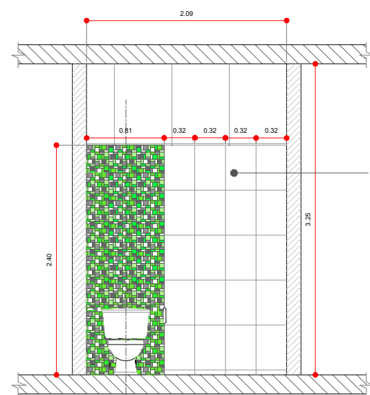
CORTE A-A
