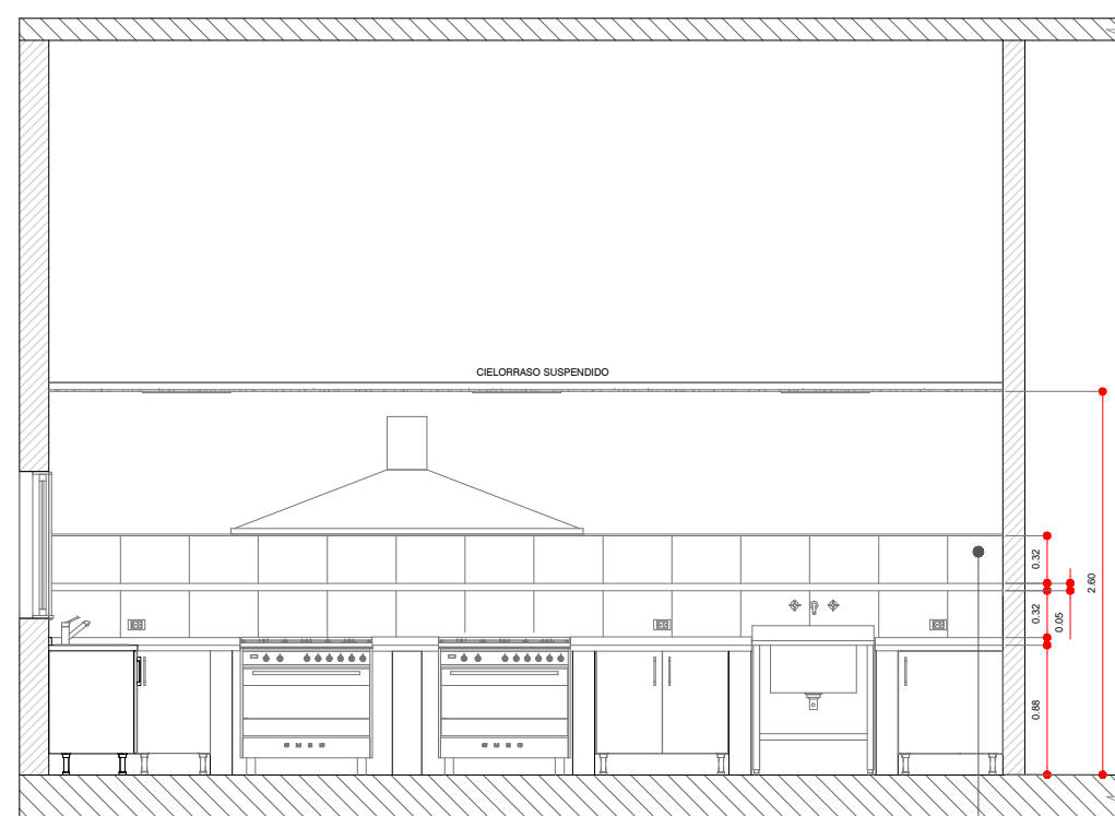
CORTE A-A
