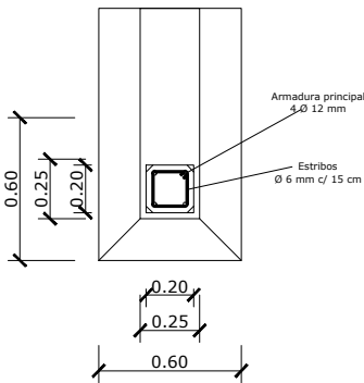
DETALLE ARMADURA DE TRONCO DE COLUMNA
