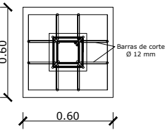
DETALLE ARMADURA DE TRONCO DE COLUMNA
