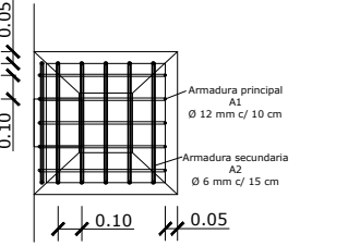
DETALLE ARMADURA DE BASE
