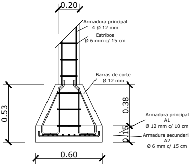
DETALLE ARMADURA CORTE
