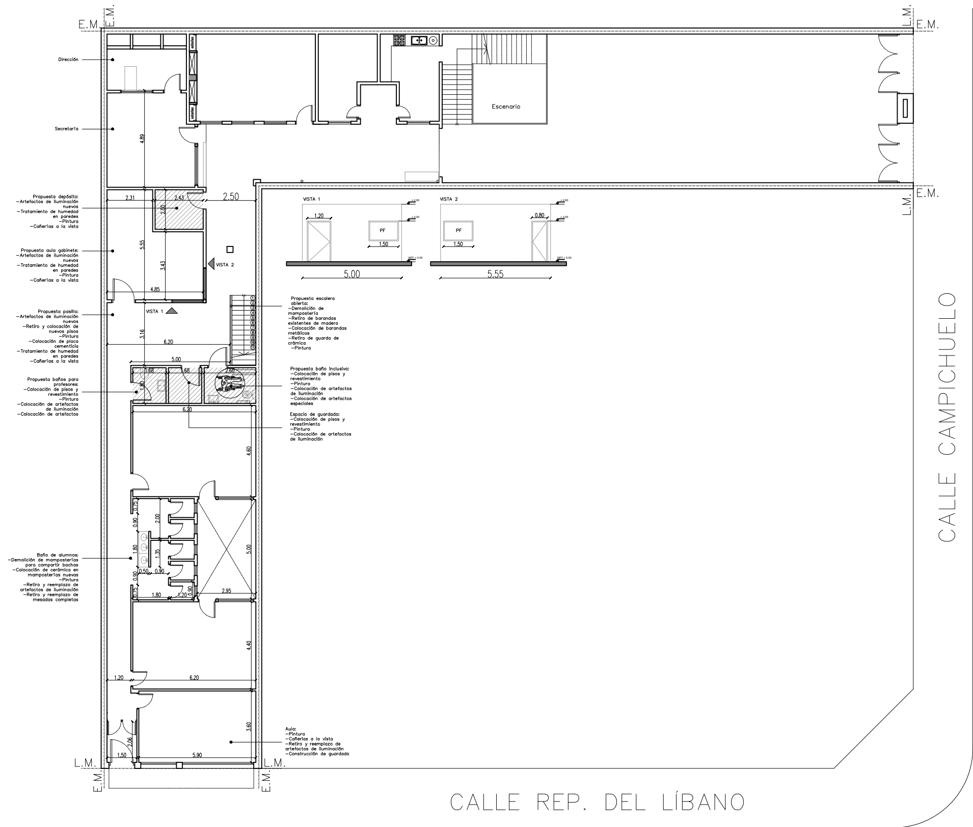
PLANTA BAJA
