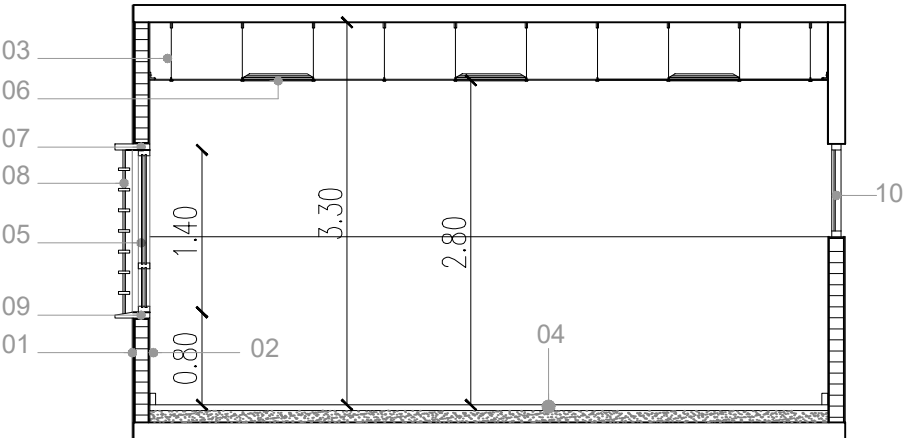
CORTE AULA
