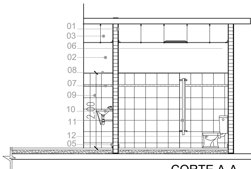
CORTE A-A
