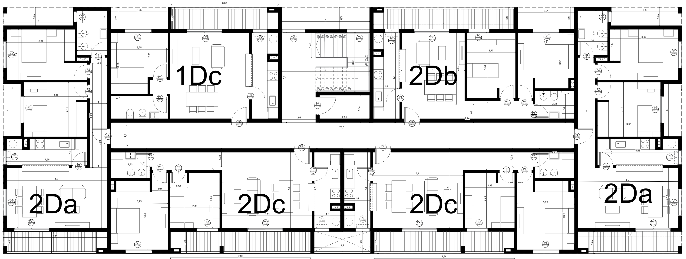
PLANTA TIPO
