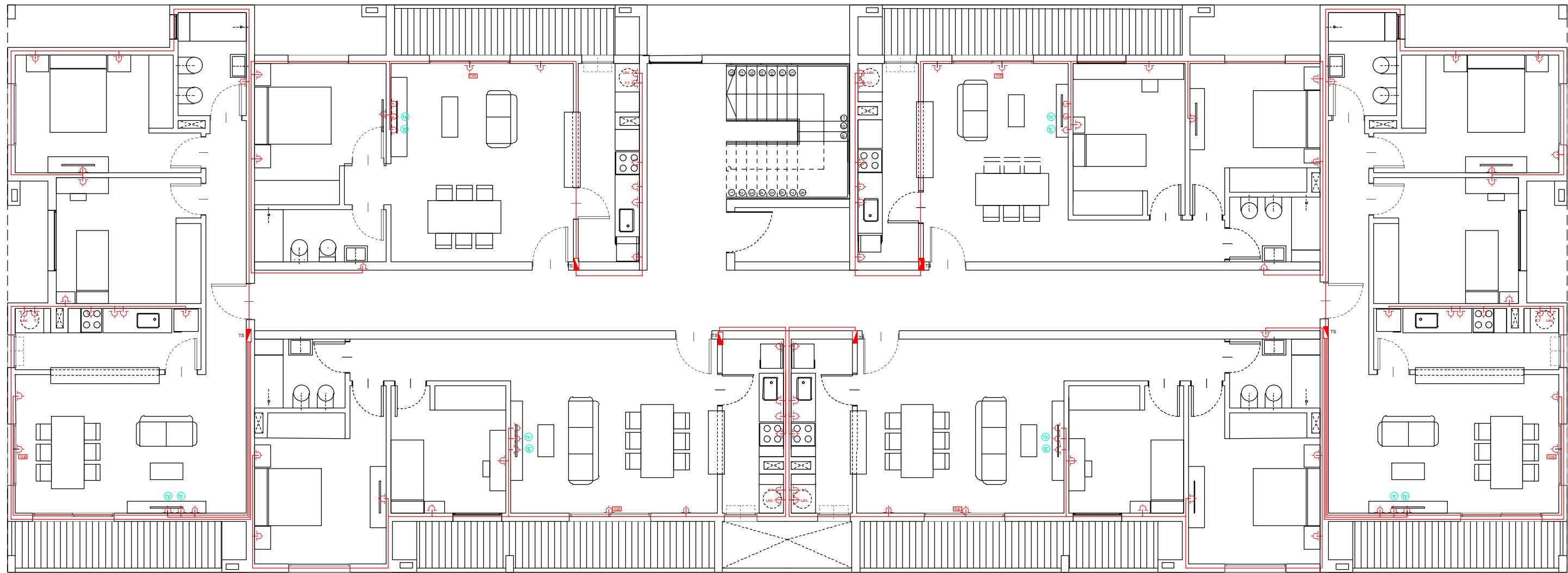
PLANTA TIPO
