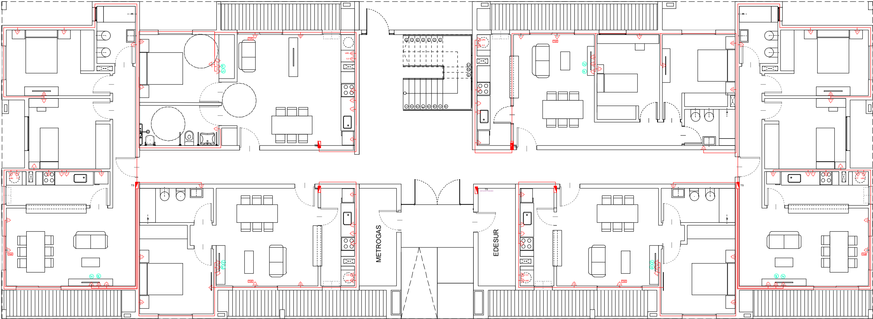
PLANTA BAJA
