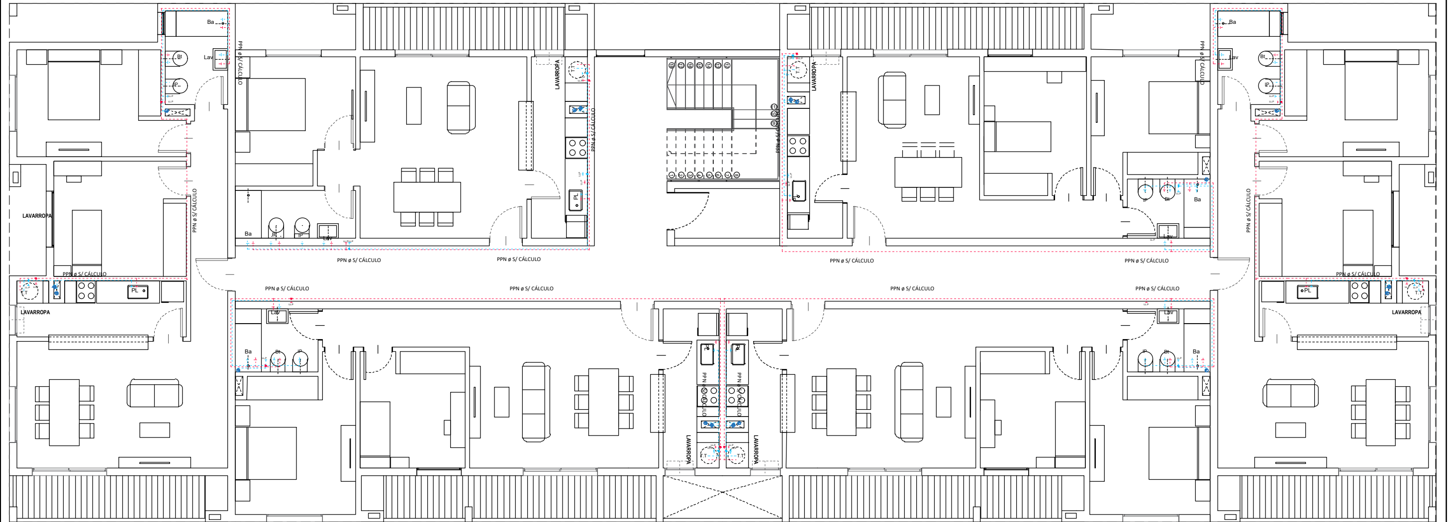
PLANTA TIPO
