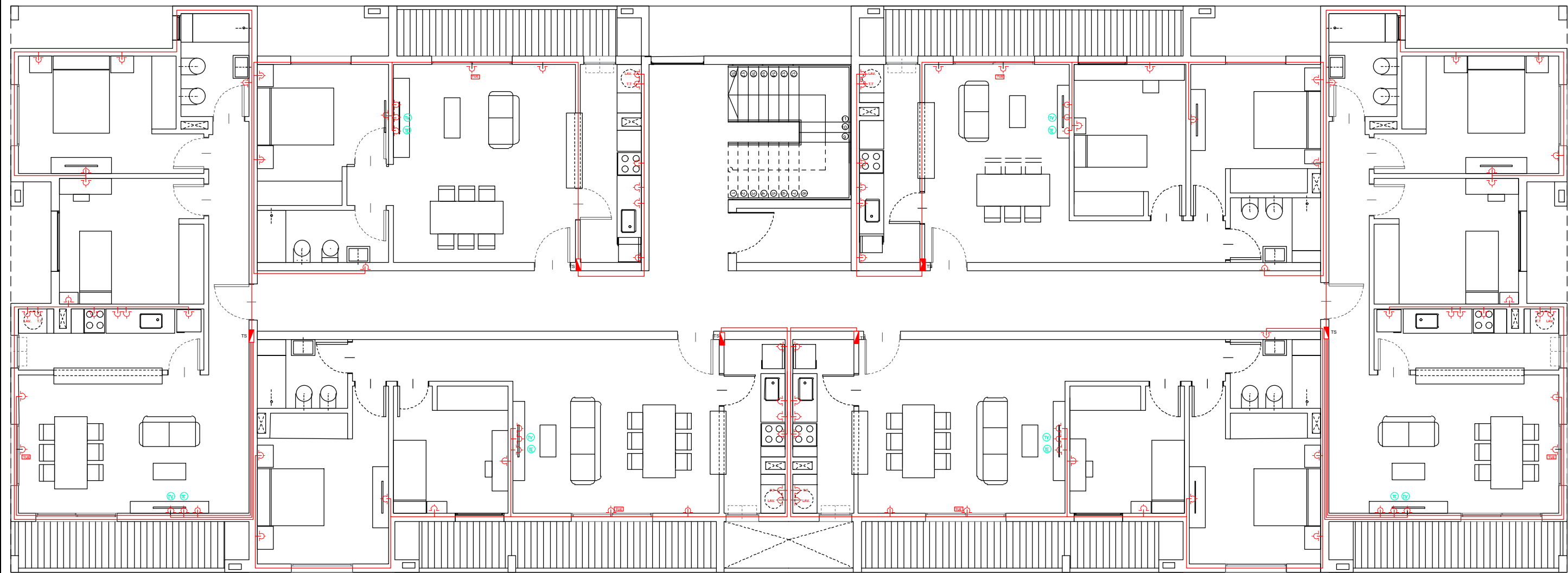
PLANTA TIPO
