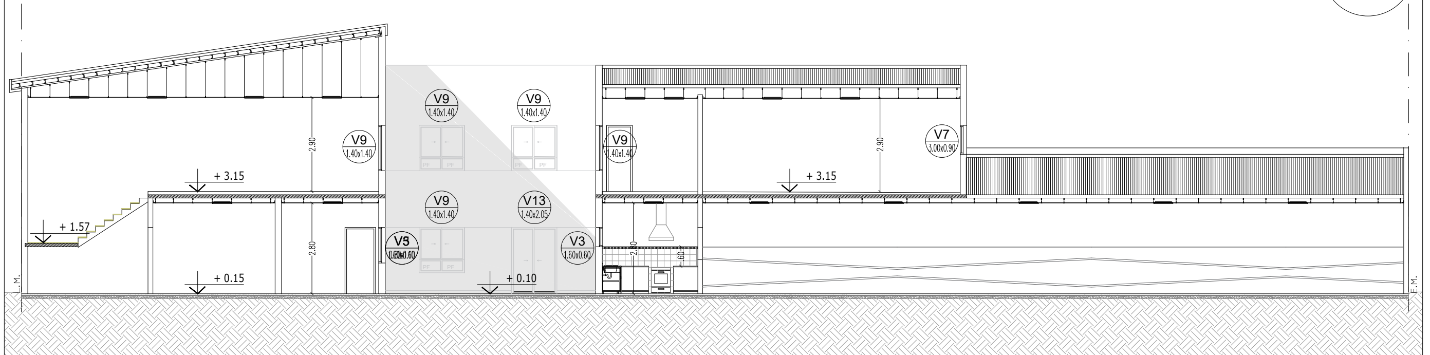
CORTE A-Á
