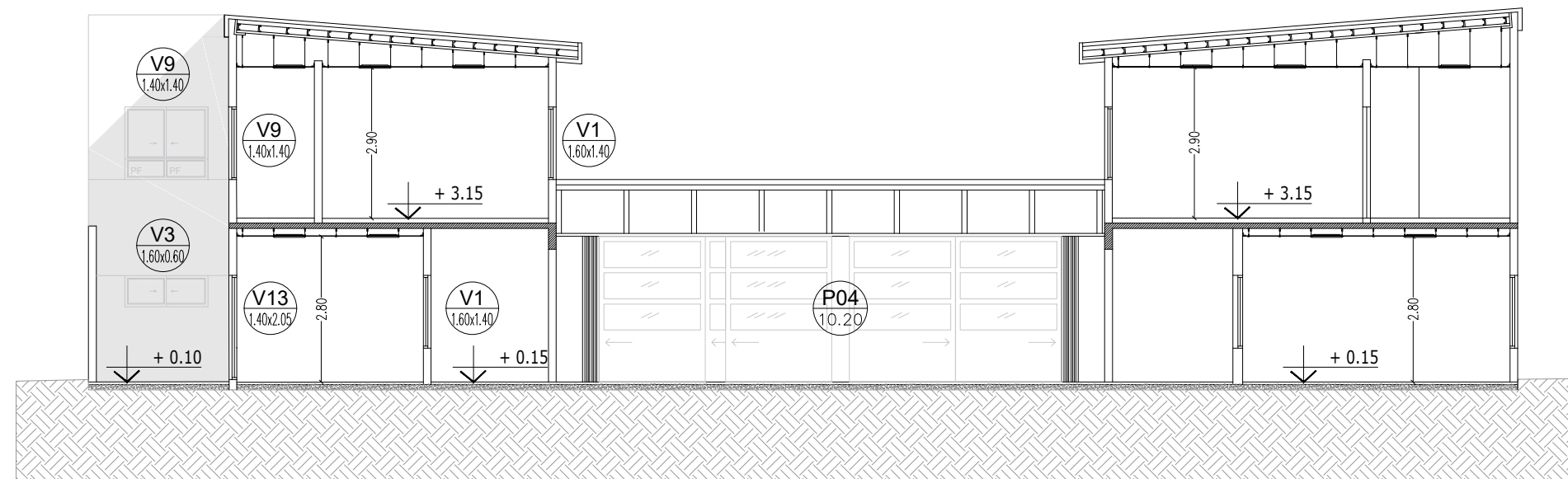
CORTE B-B
