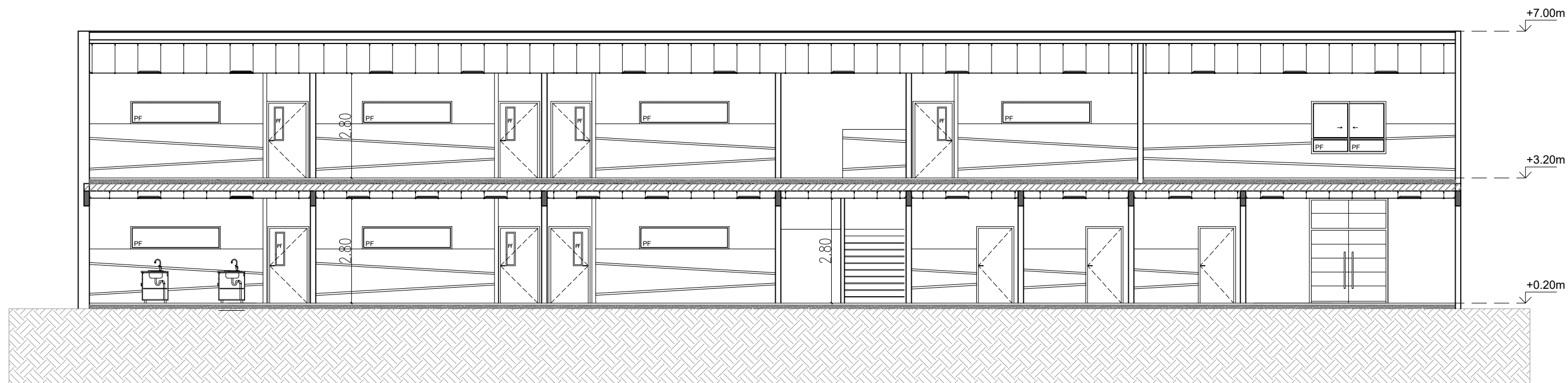
CORTE C-C
