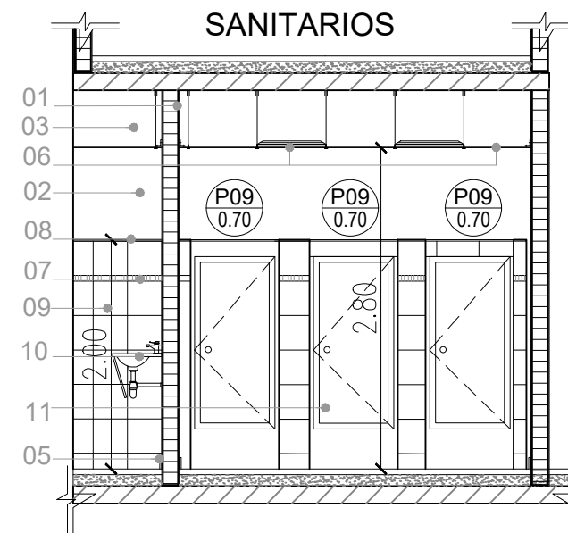
CORTE B-B
