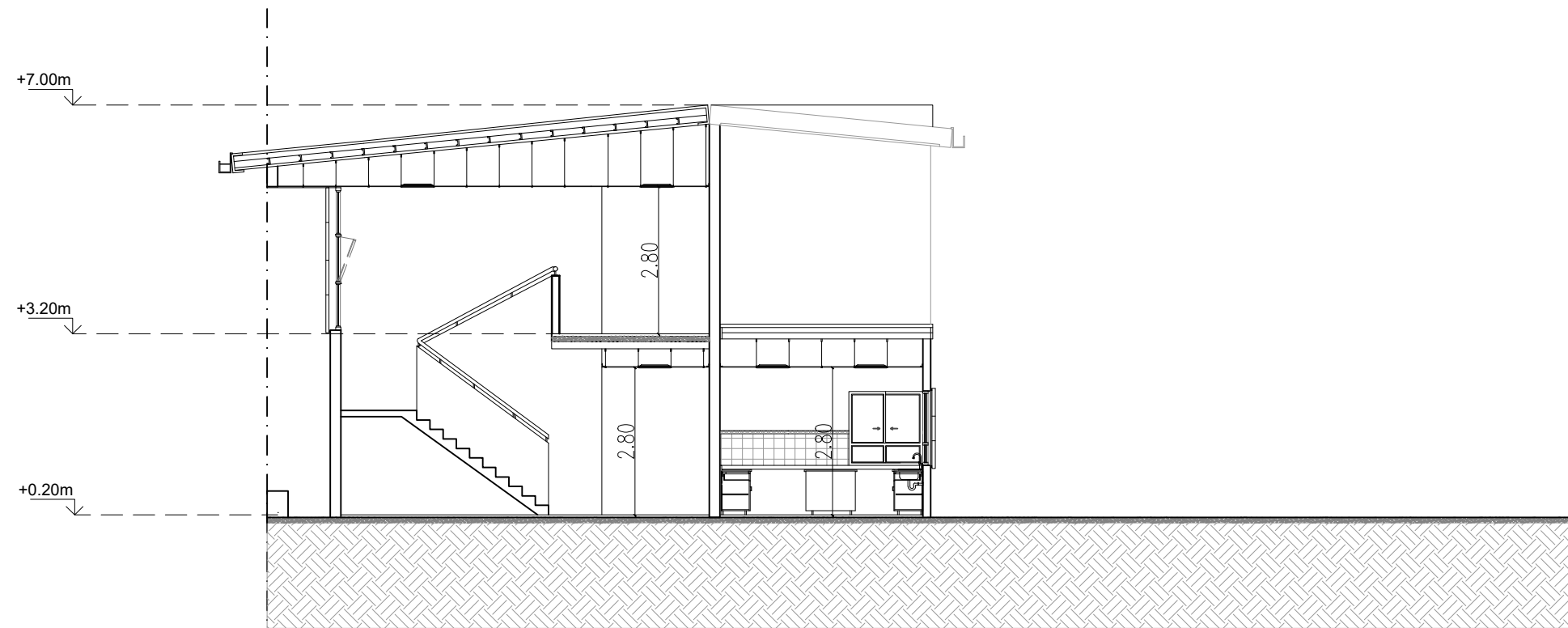
CORTE B-B
