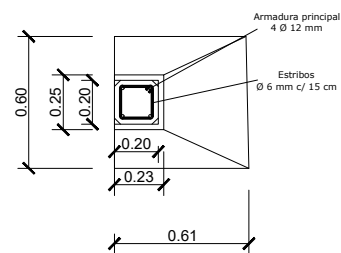
DETALLE ARMADURA DE TRONCO DE COLUMNA
