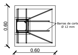
DETALLE ARMADURA DE TRONCO DE COLUMNA
