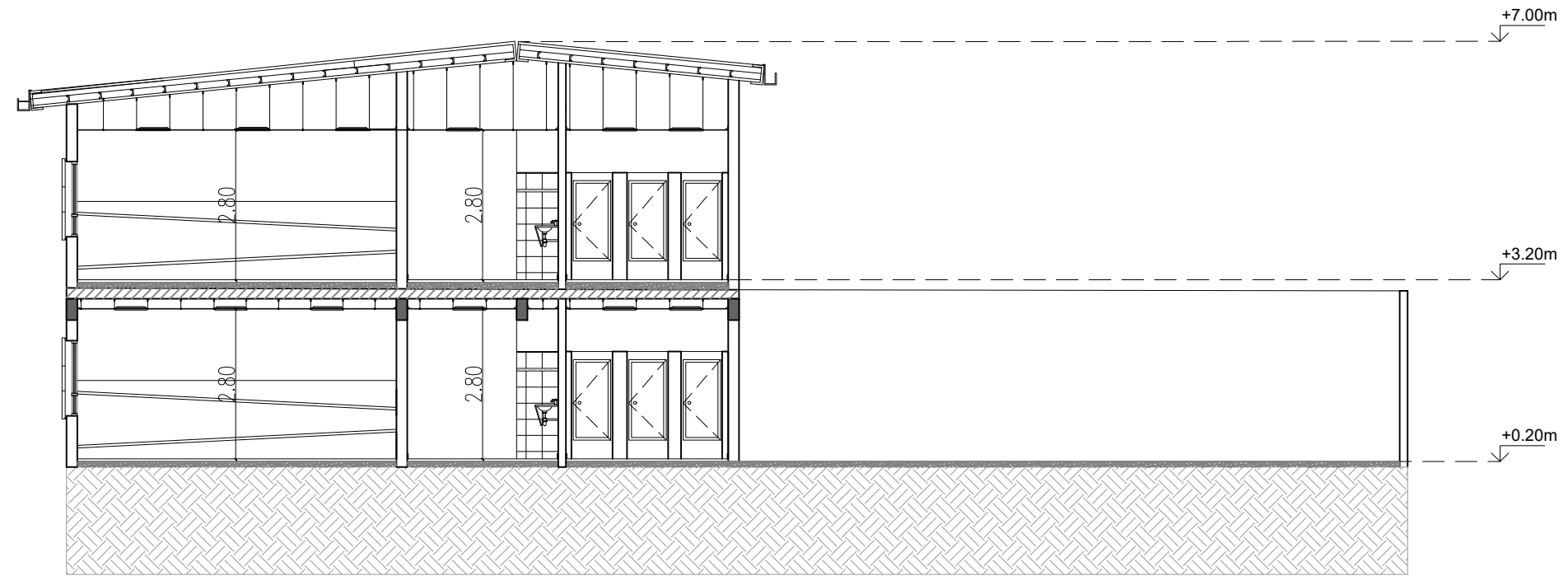
CORTE A-A
