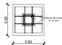
DETALLE ARMADURA DE TRONCO DE COLUMNA
