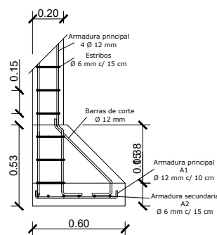
DETALLE ARMADURA CORTE
