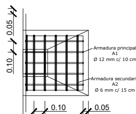
DETALLE ARMADURA DE BASE
