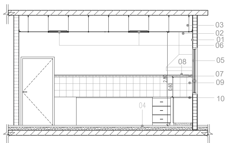
CORTE A-A
