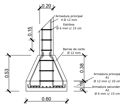
DETALLE ARMADURA CORTE
