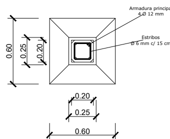
DETALLE ARMADURA DE TRONCO DE COLUMNA
