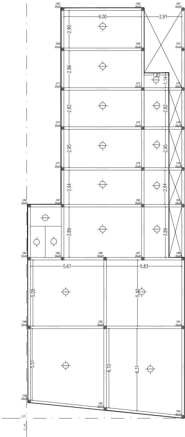
ESTRUCTURA SOBRE PLANTA BAJA
