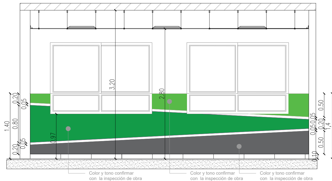
CORTE AULA
