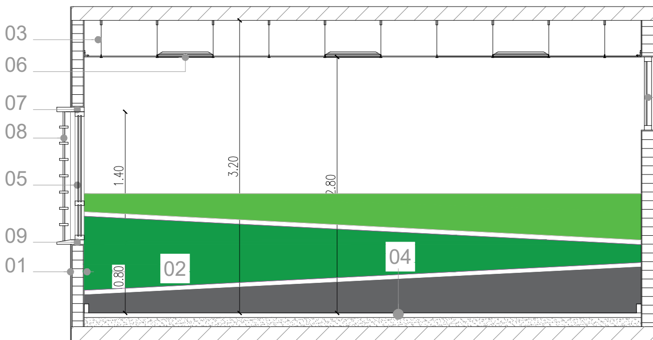
CORTE AULA
