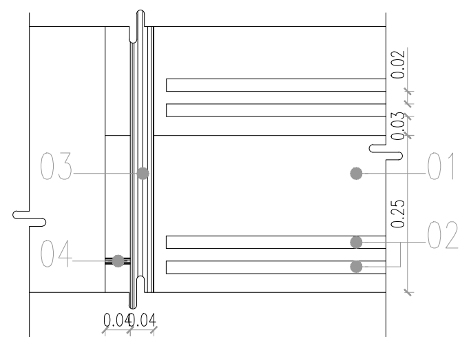
DETALLE 1
