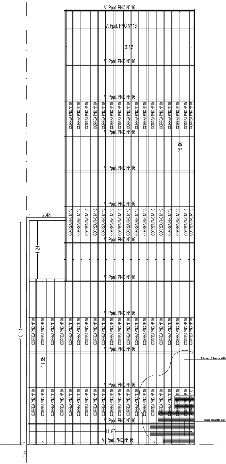
ESTRUCTURA CUBIERTA
