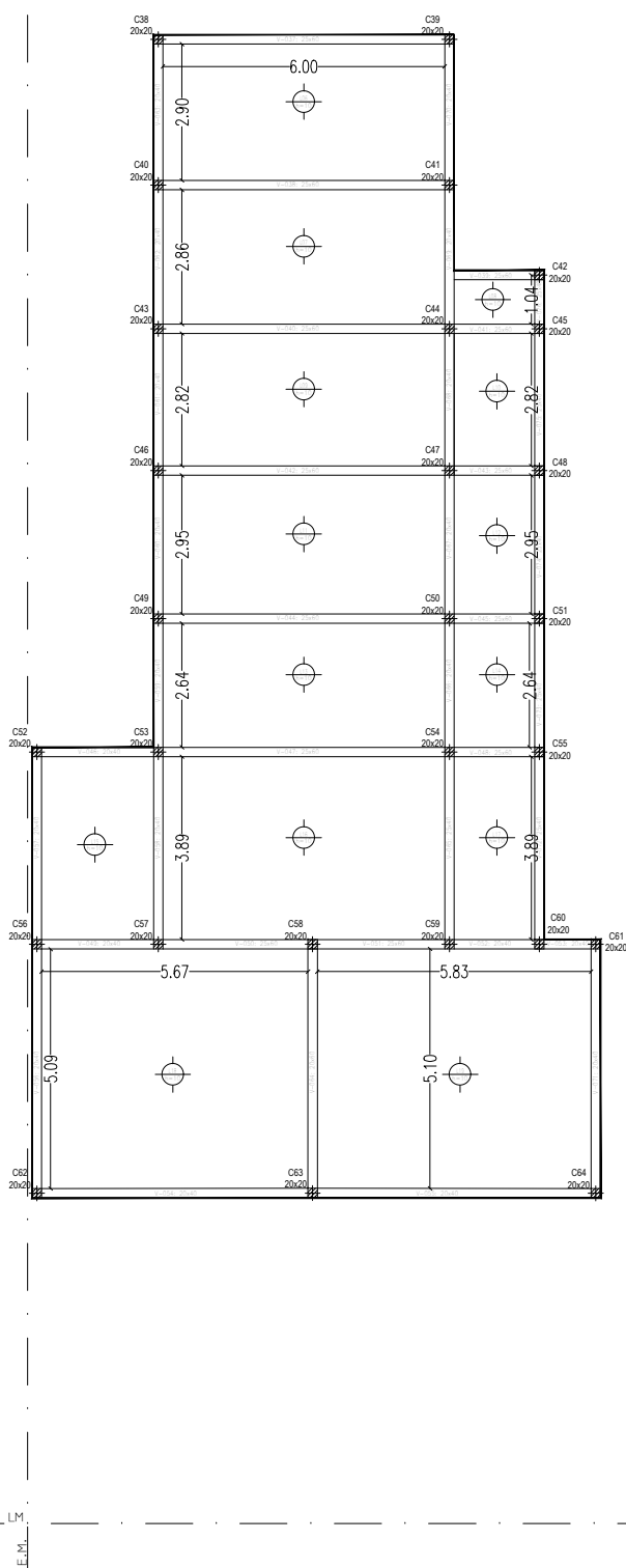
ESTRUCTURA SOBRE NIVEL +1.20m
