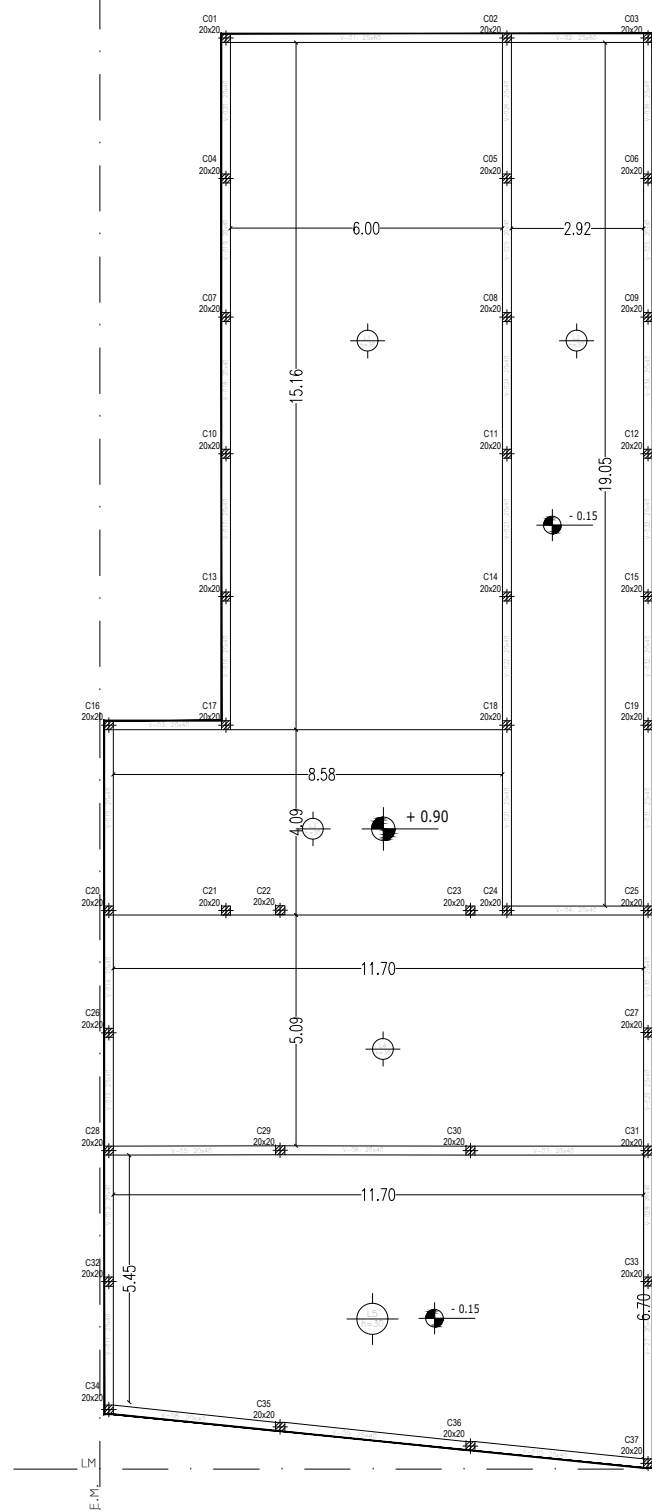
FUNDACIONES - PLATEA
