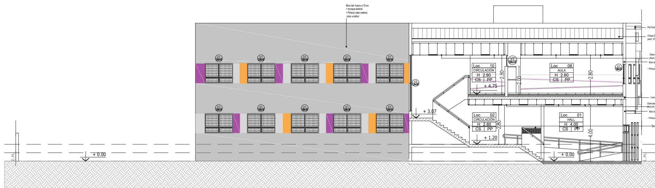
CORTE CONSTRUCTIVO B-B
