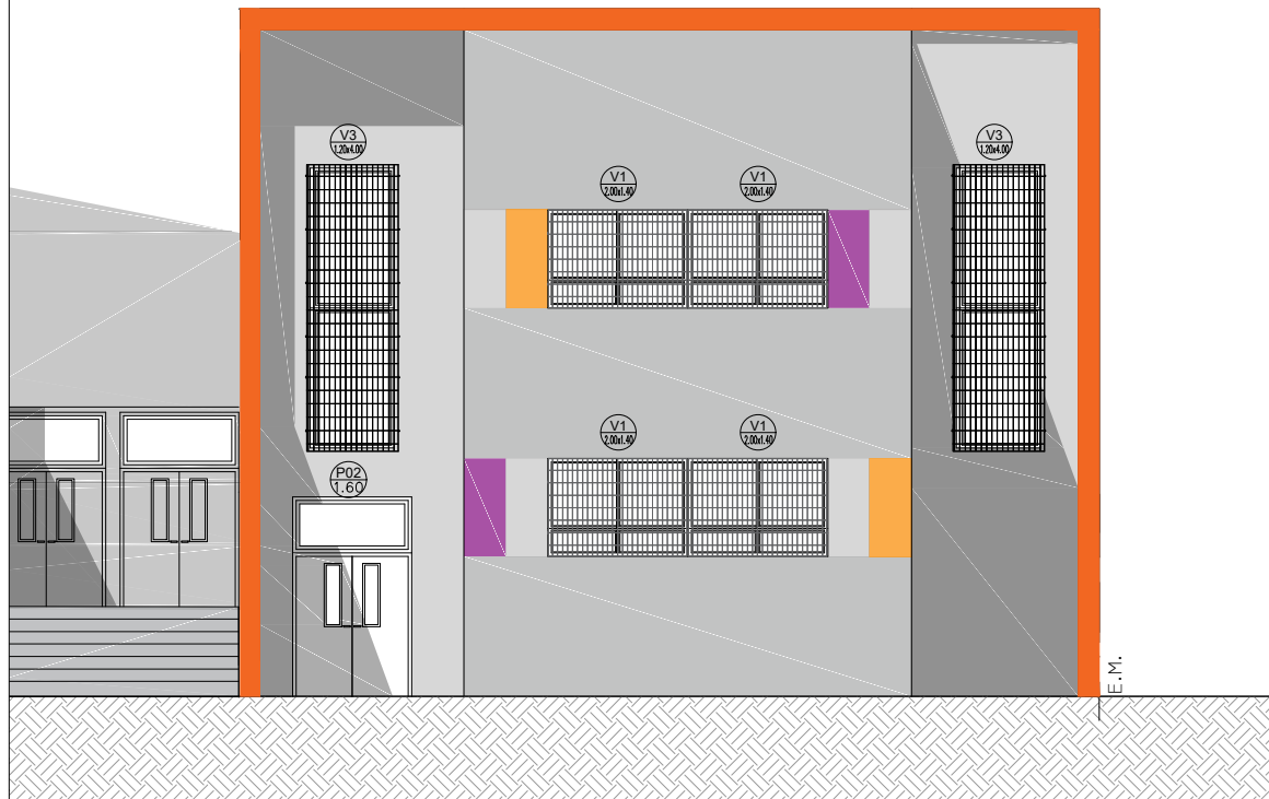
FACHADA CONTRAFRENTE
