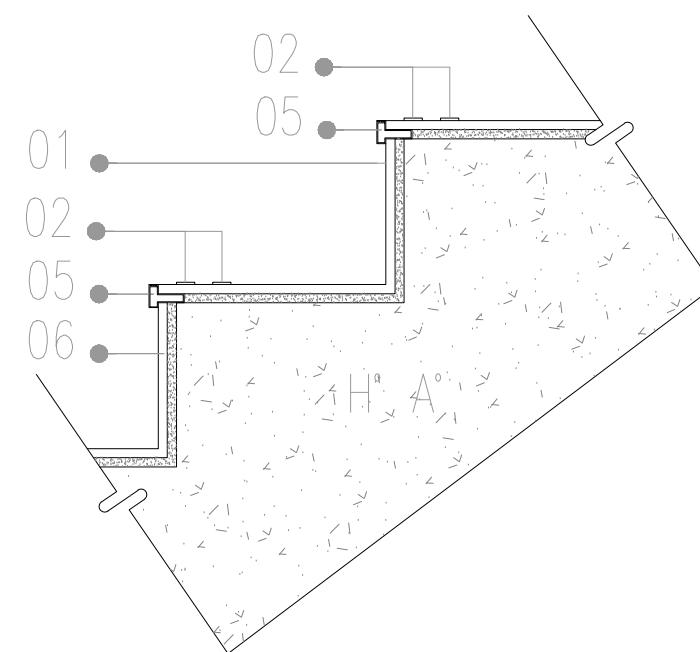
DETALLE 2
