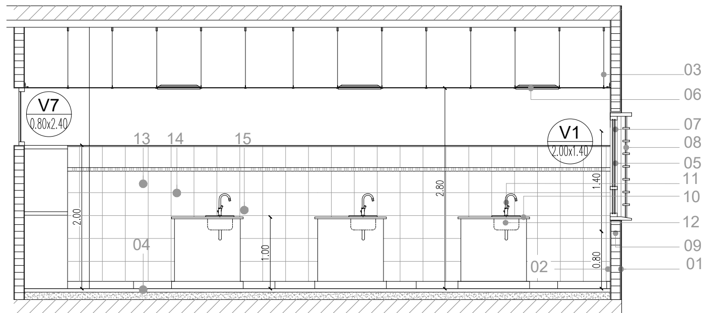
CORTE BB LABORATORIO
