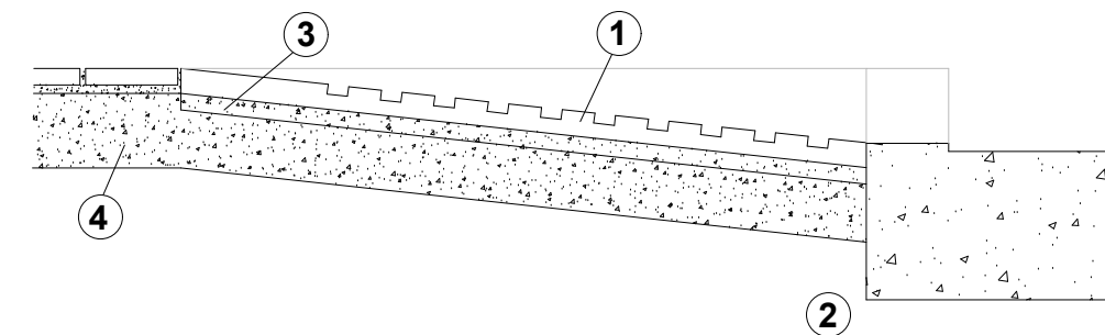
Corte ESC. 1:20
