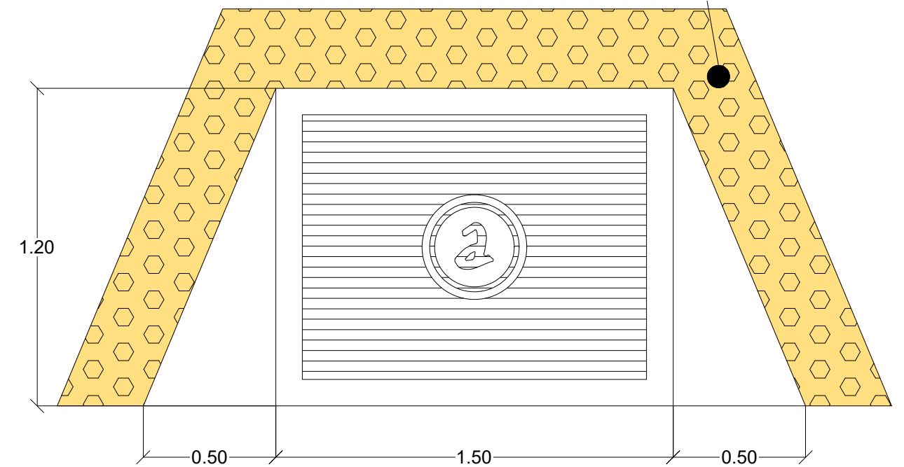
Planta Rampa Simple ESC. 1:20
