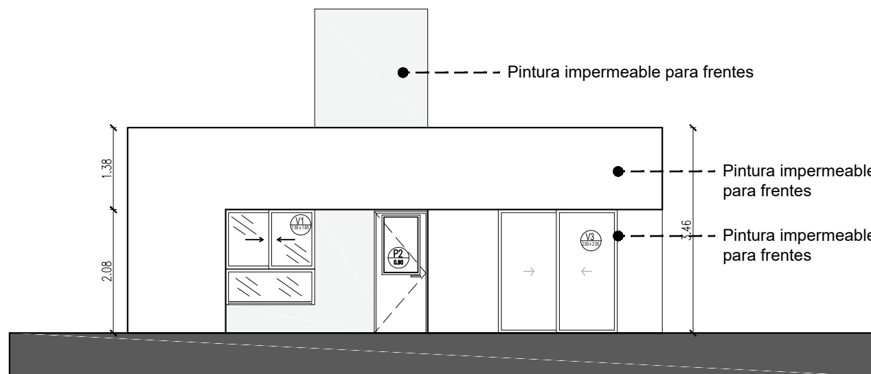
CONTRA FACHADA
