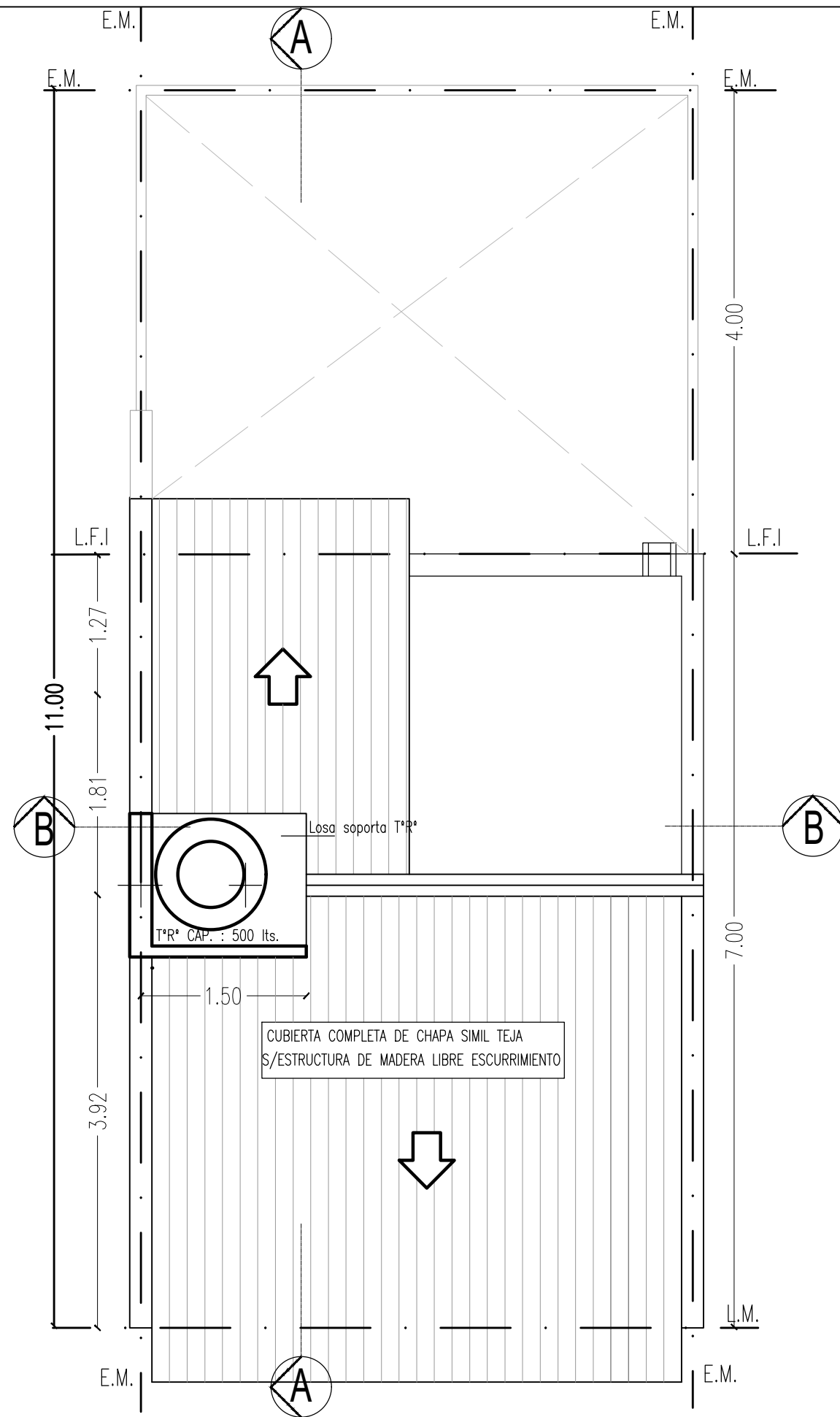
PLANTA DE TECHO
