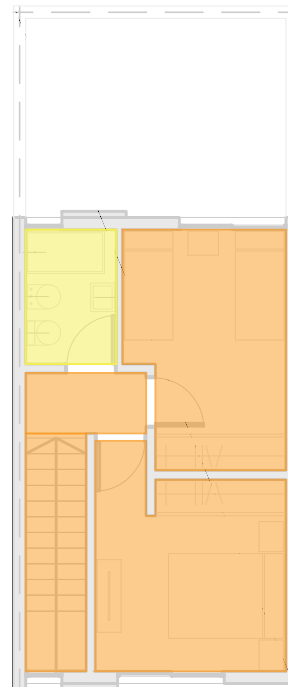
PLANTA ALTA
