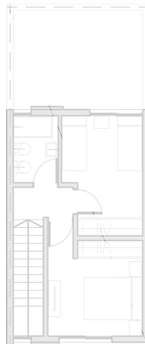
PLANTA ALTA
