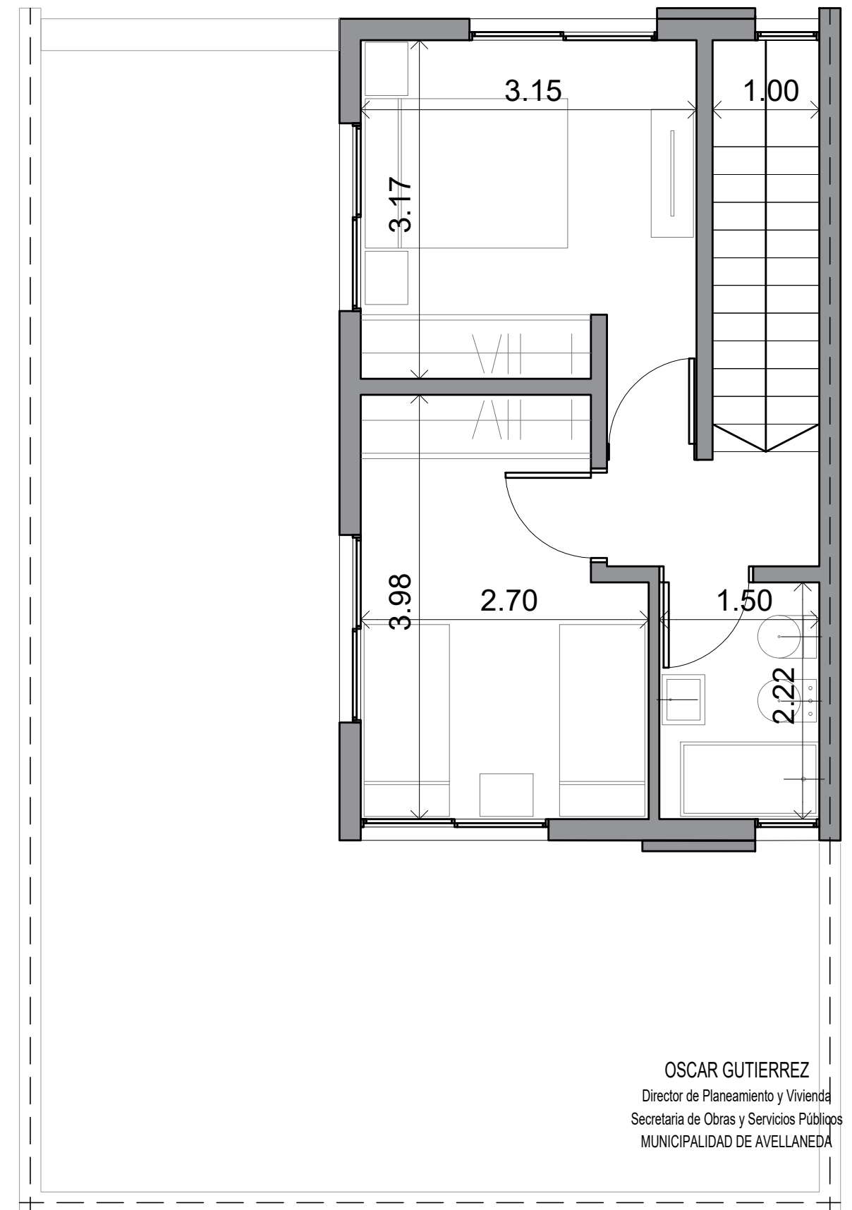
PLANTA ALTA
