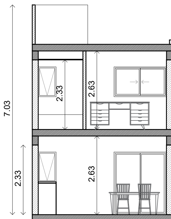
CORTE A-A
