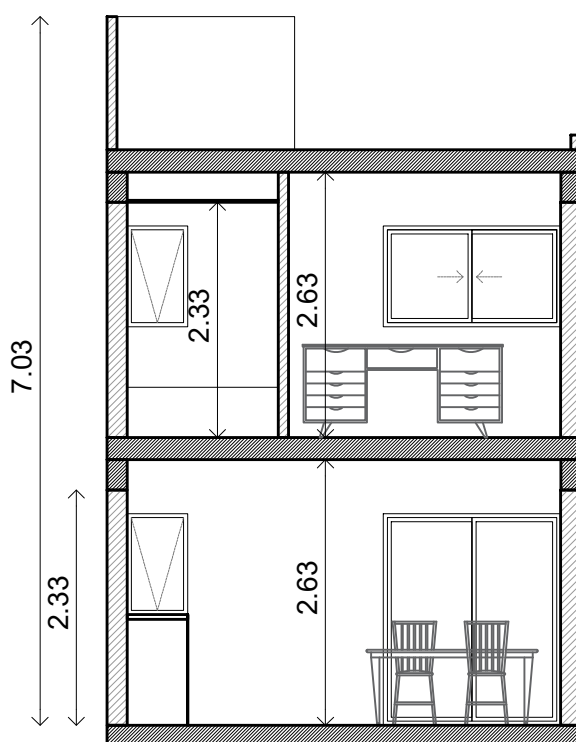
CORTE A-A
