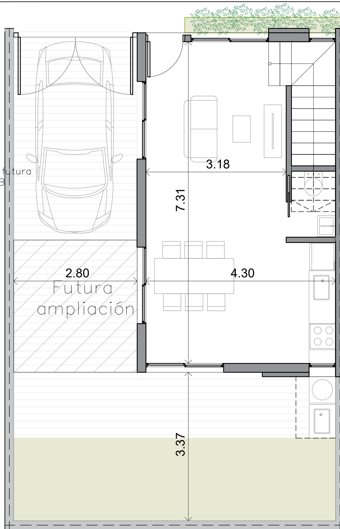
PLANTA BAJA
