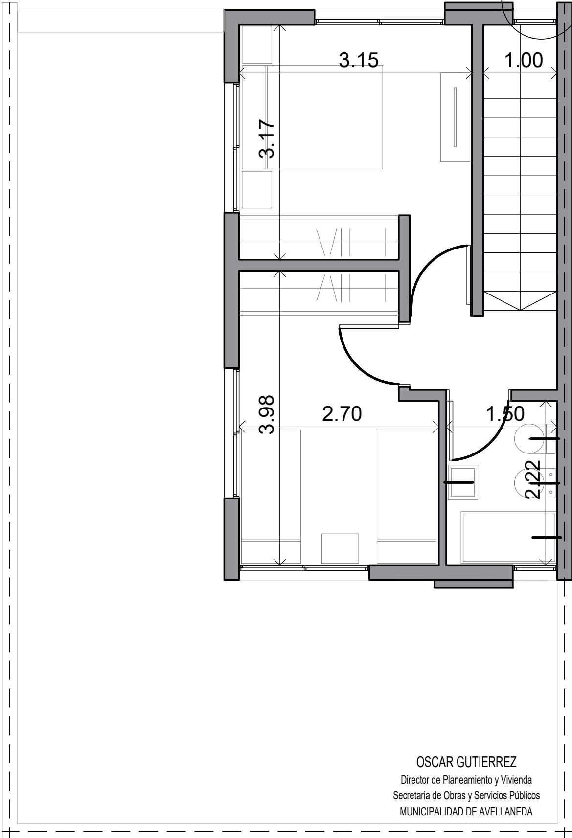
PLANTA ALTA
