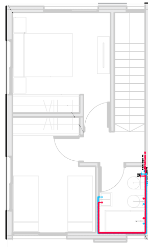
PLANTA ALTA
