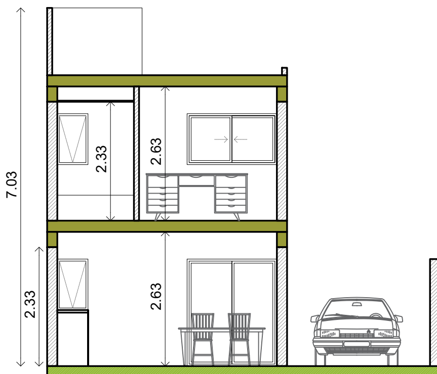
CORTE
