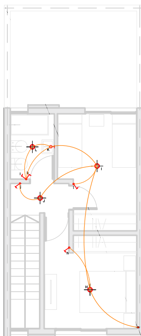
PLANTA ALTA
