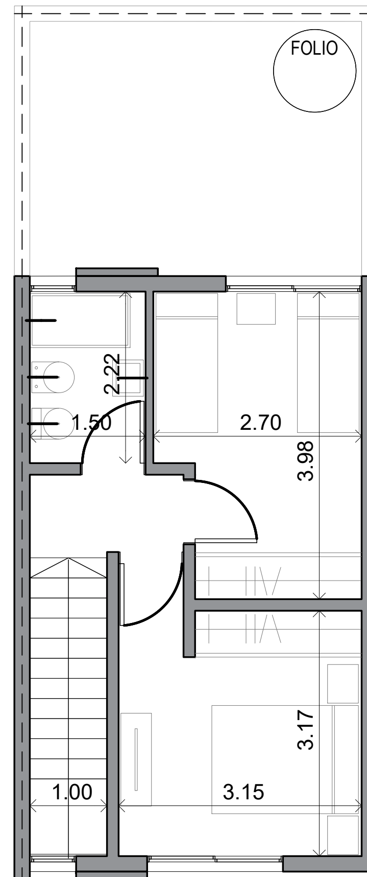
PLANTA ALTA
