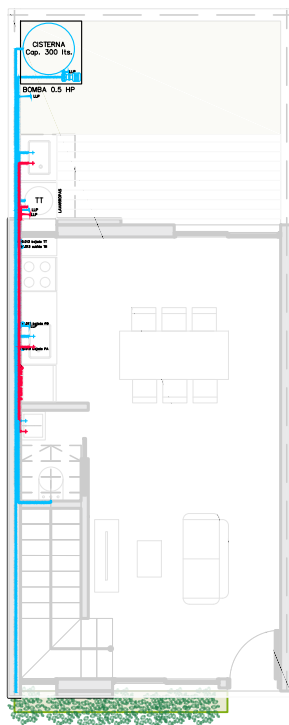
PLANTA BAJA
