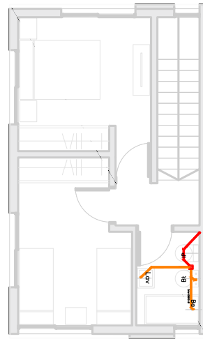
PLANTA ALTA
