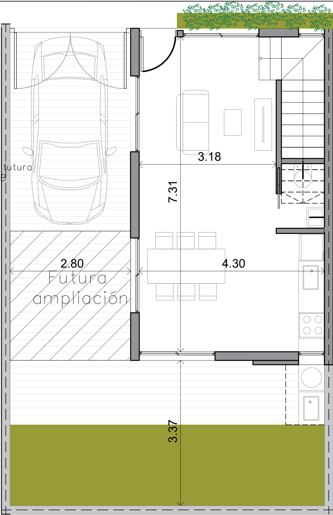
PLANTA BAJA
