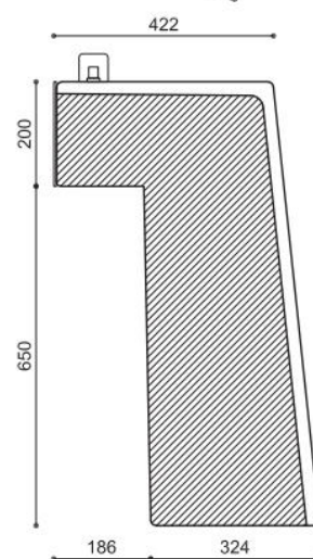
CORTE
