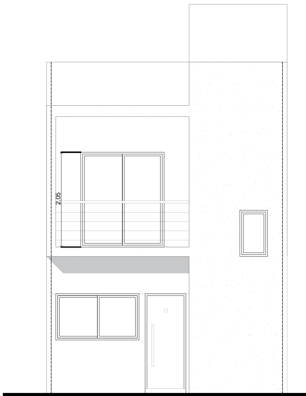
VISTA FRENTE
