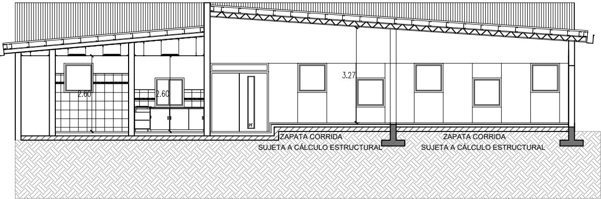
CORTE B-B
