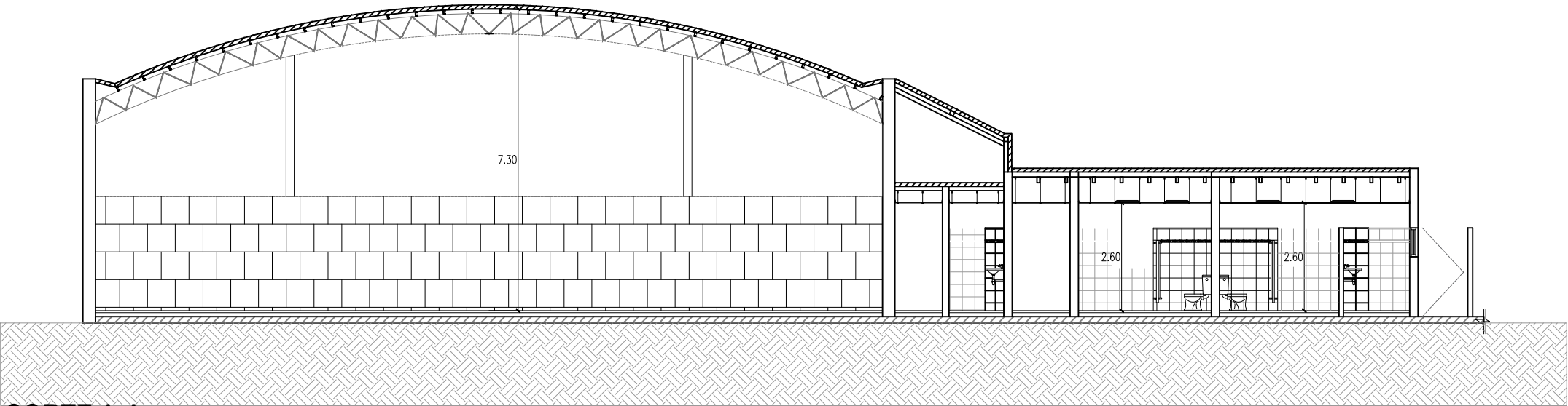
CORTE A-A
