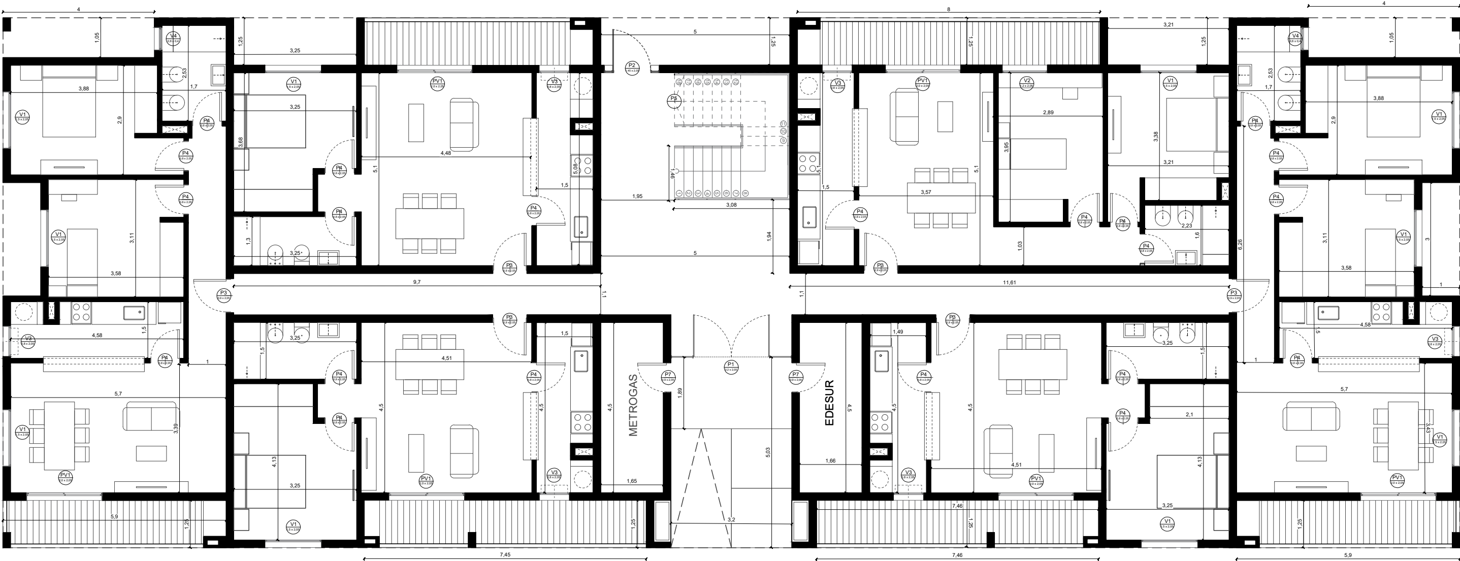
PLANTA BAJA
