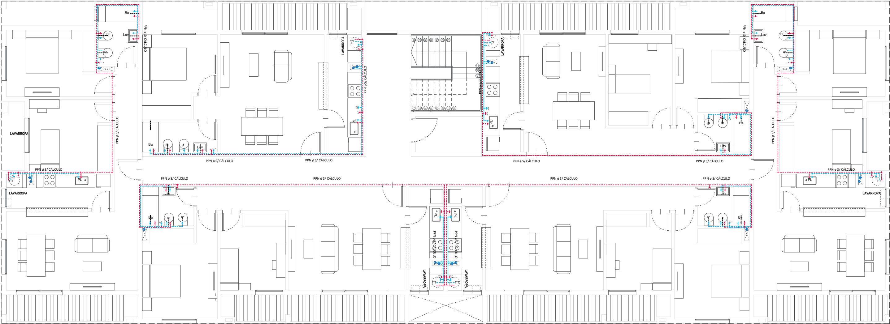
PLANTA TIPO
