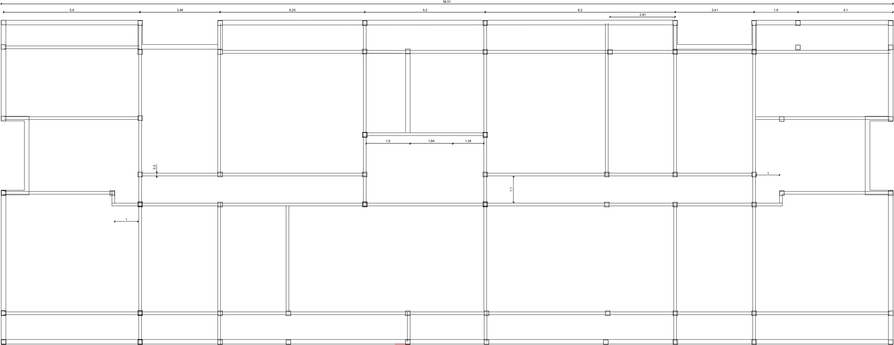
PLATEA DE FUNDACIÓN
