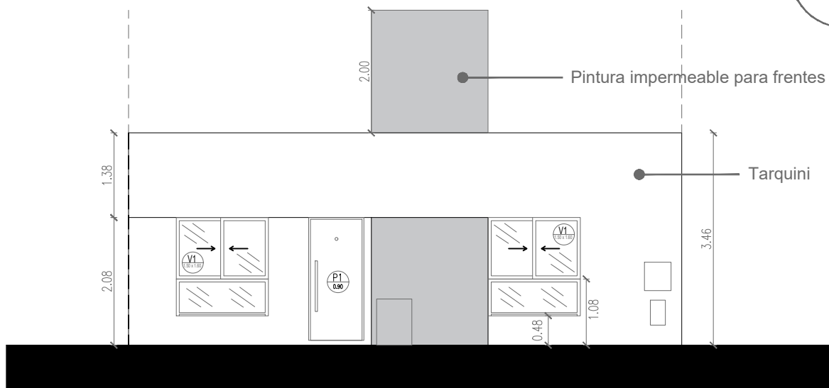
FACHADA
