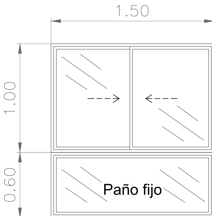
VISTA
