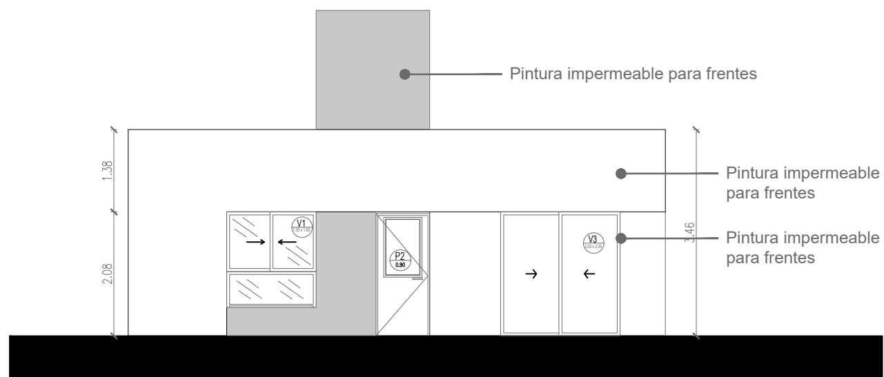
CONTRA FACHADA
