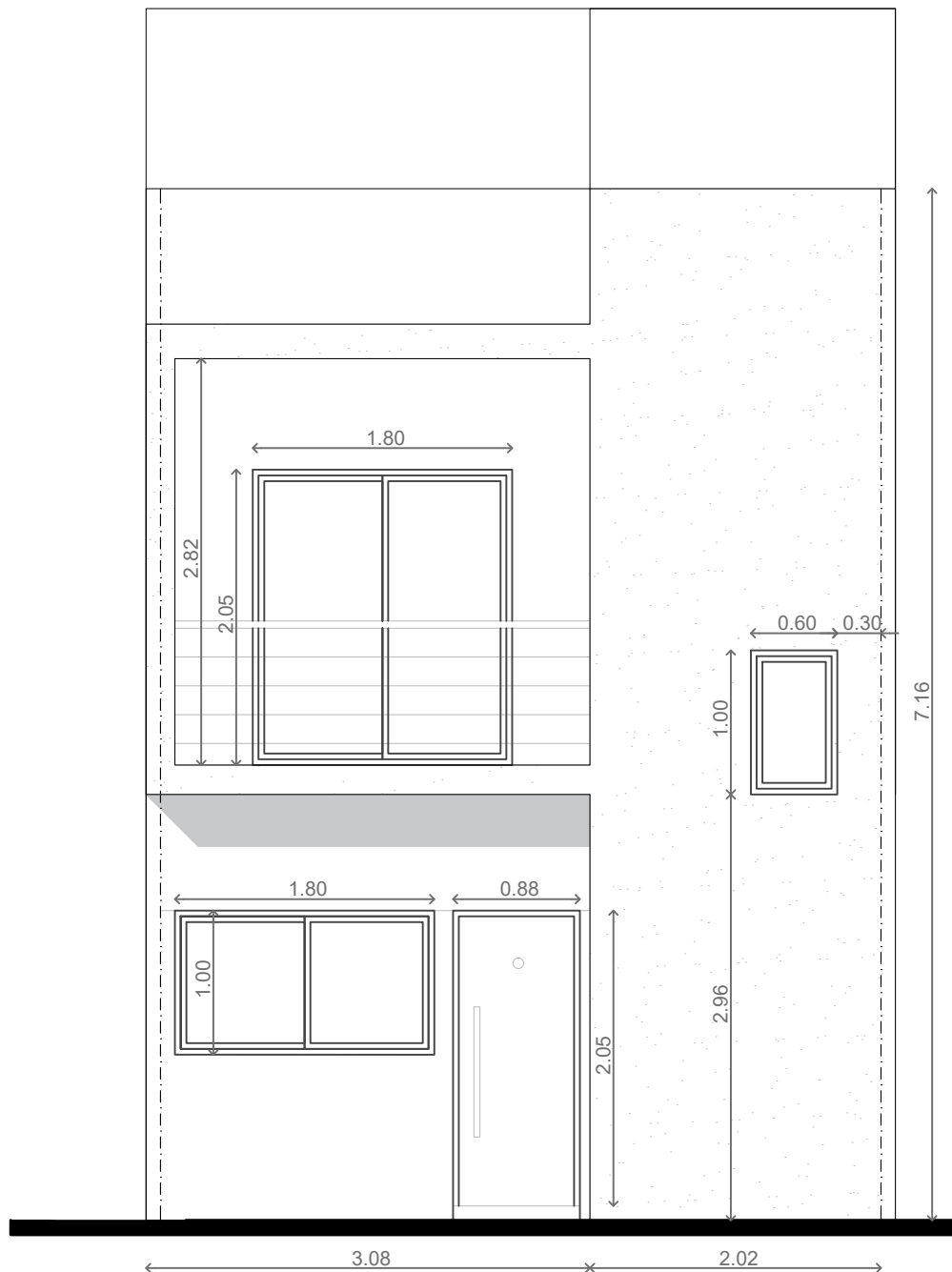
VISTA FRENTE
