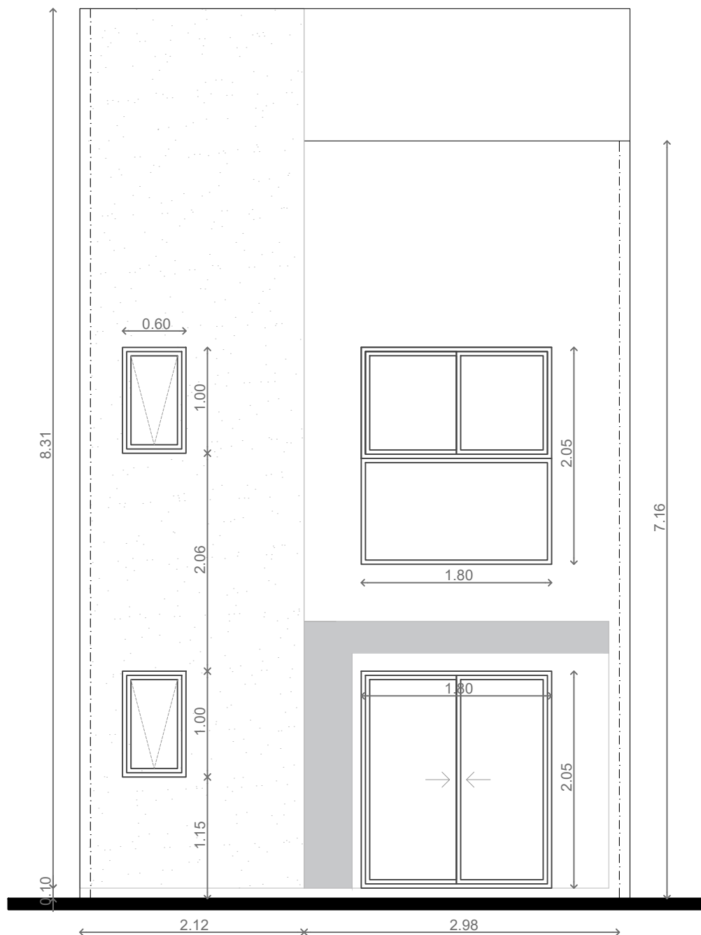
VISTA CONTRAFRENTE
