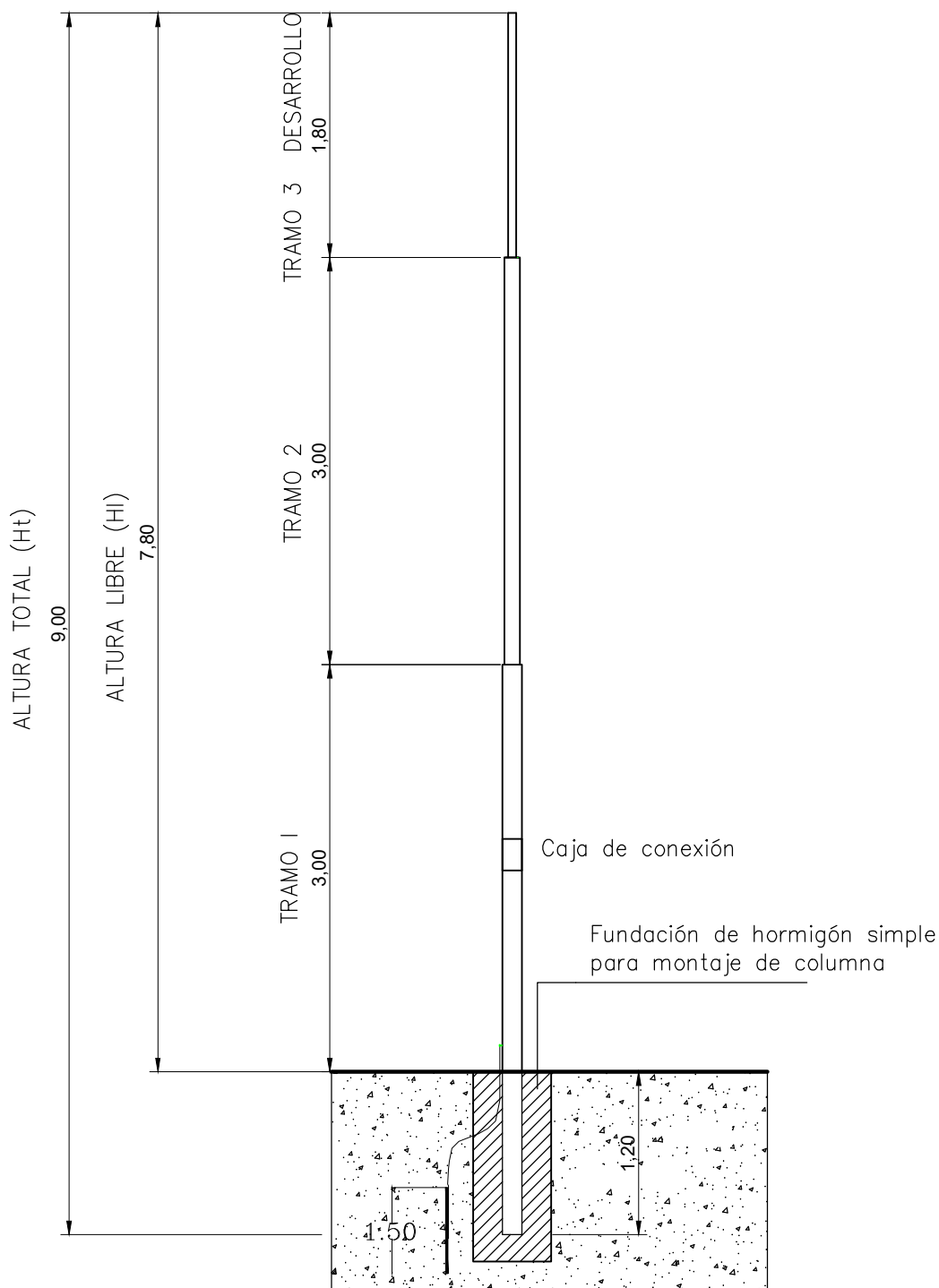
Vista lateral
