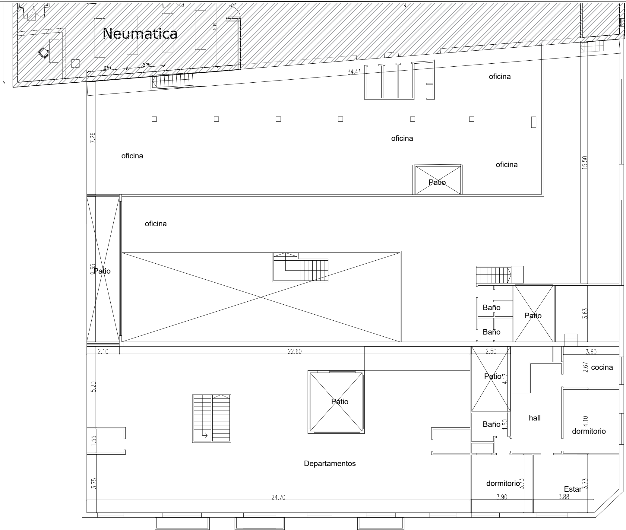
PRIMER PISO
