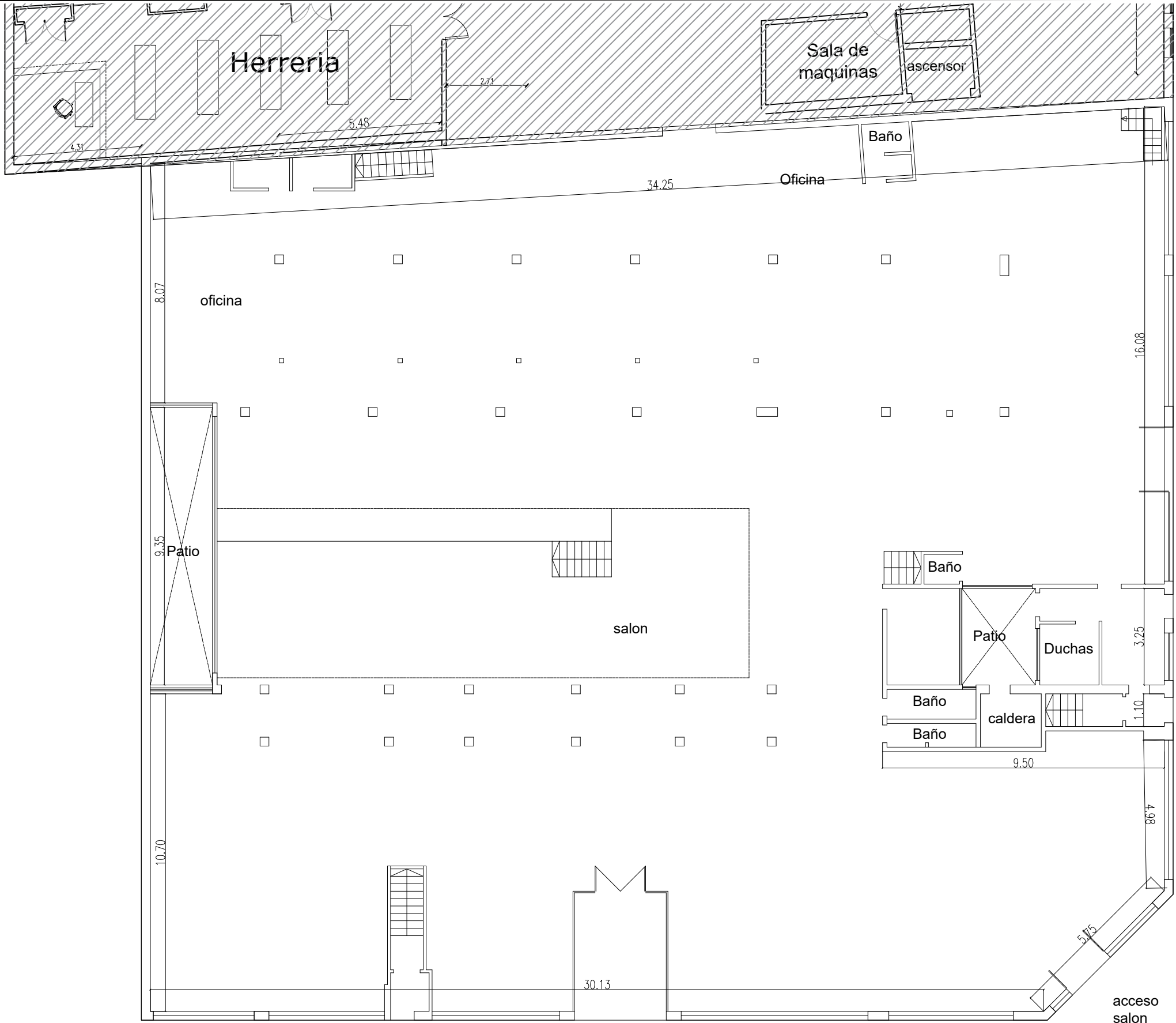
PLANTA BAJA
