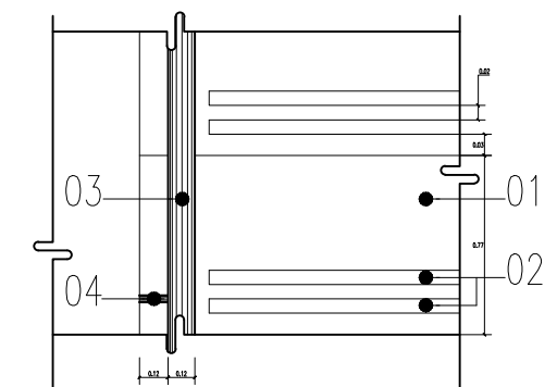
DETALE 1
