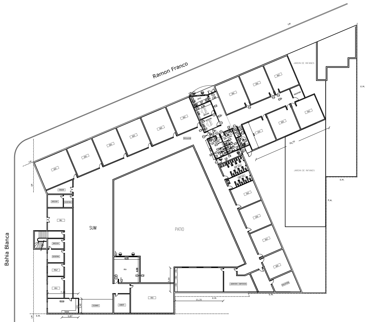
PLANTA BAJA
