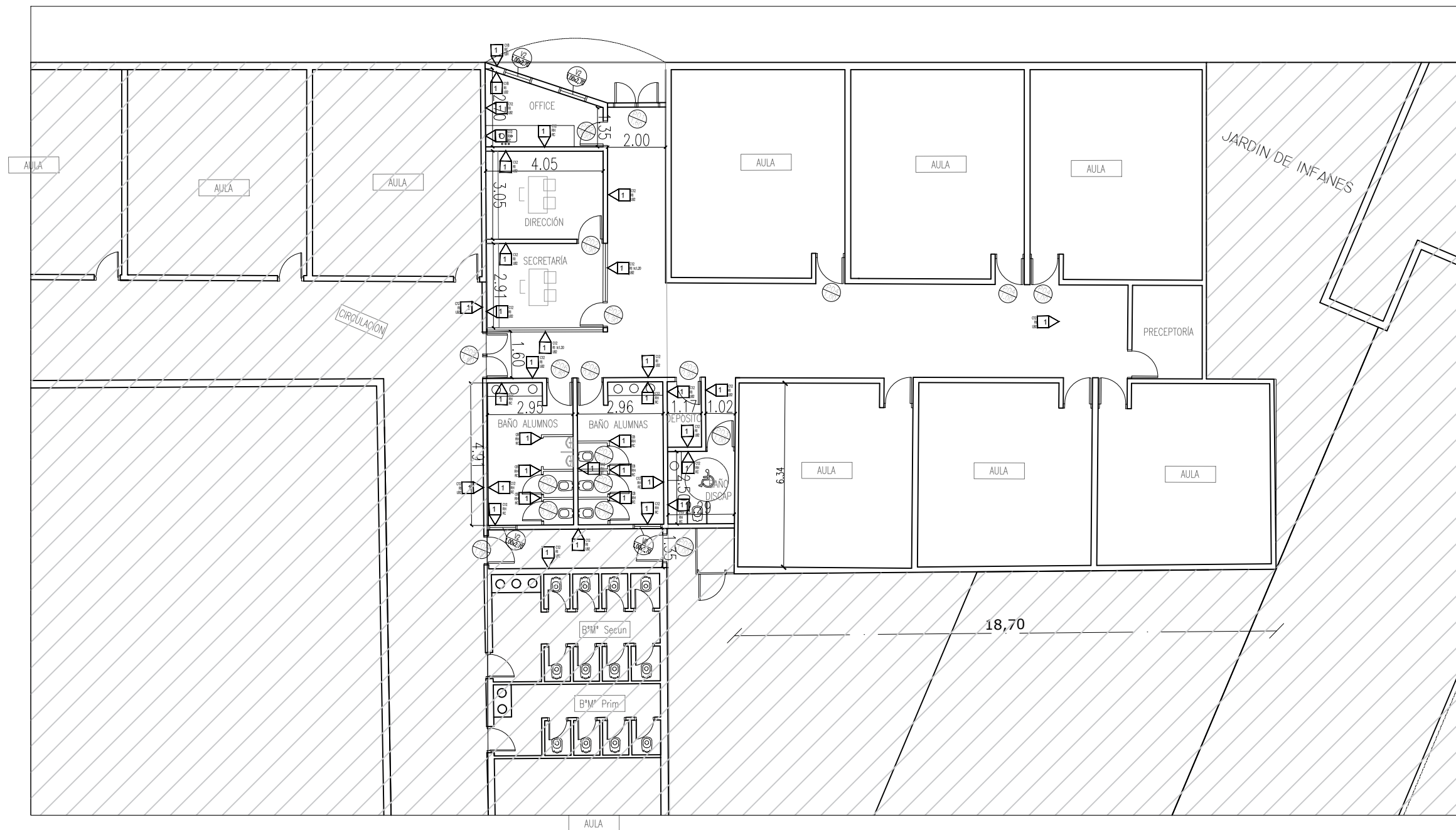
PLANTA BAJA
