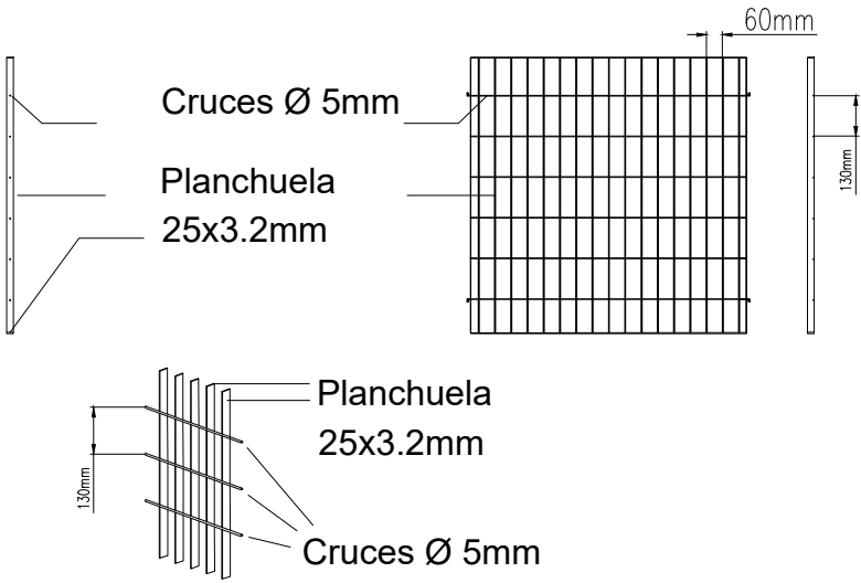
Reja techno tipo TDL planchuela 25x3.2 mm cruces Ø 5mm
