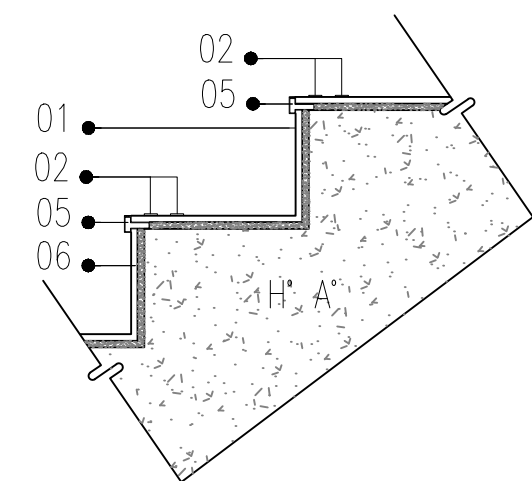
DETALLE 2
