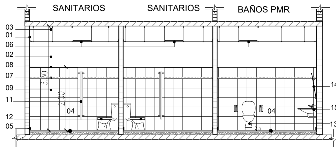
CORTE A-A
