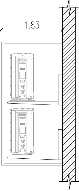
VISTA LATERAL
