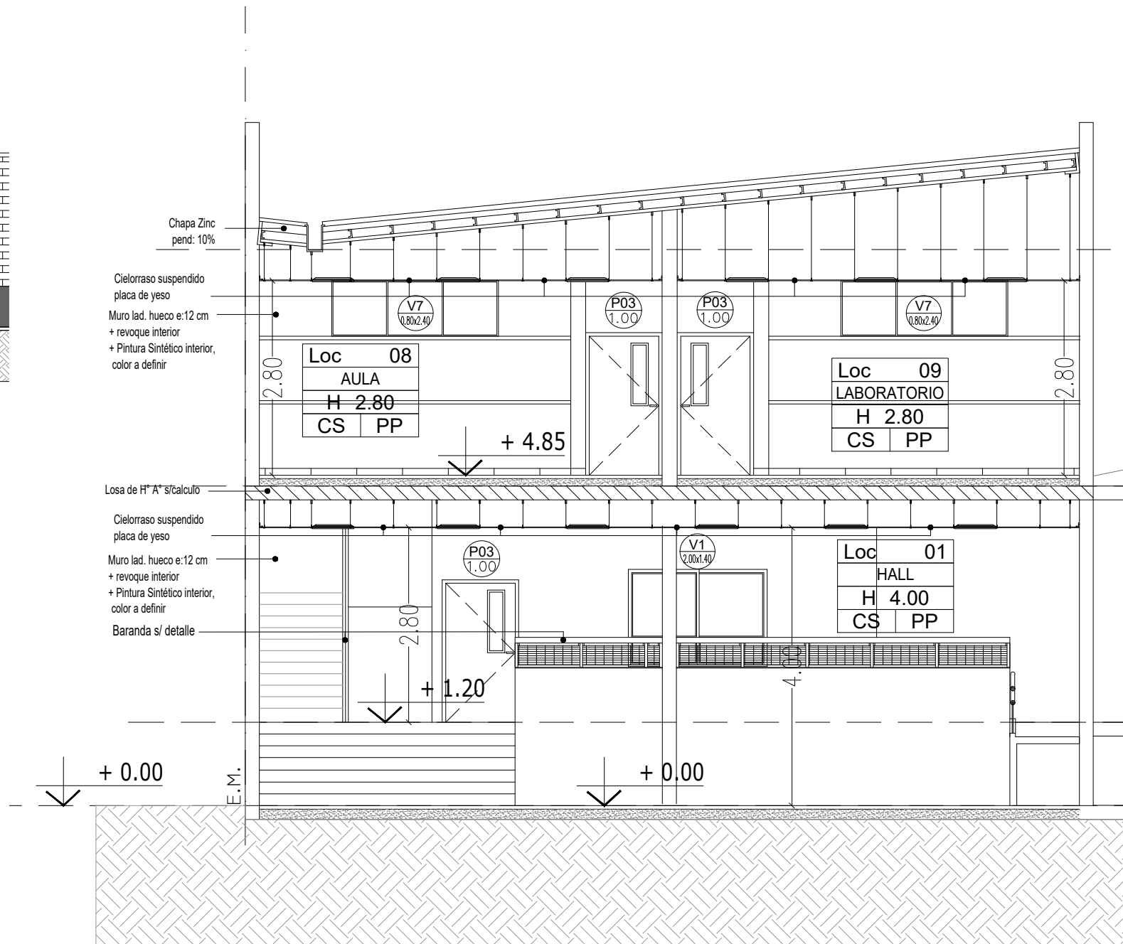
CORTE CONSTRUCTIVO A-A
