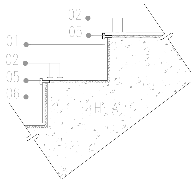
DETALLE 2
