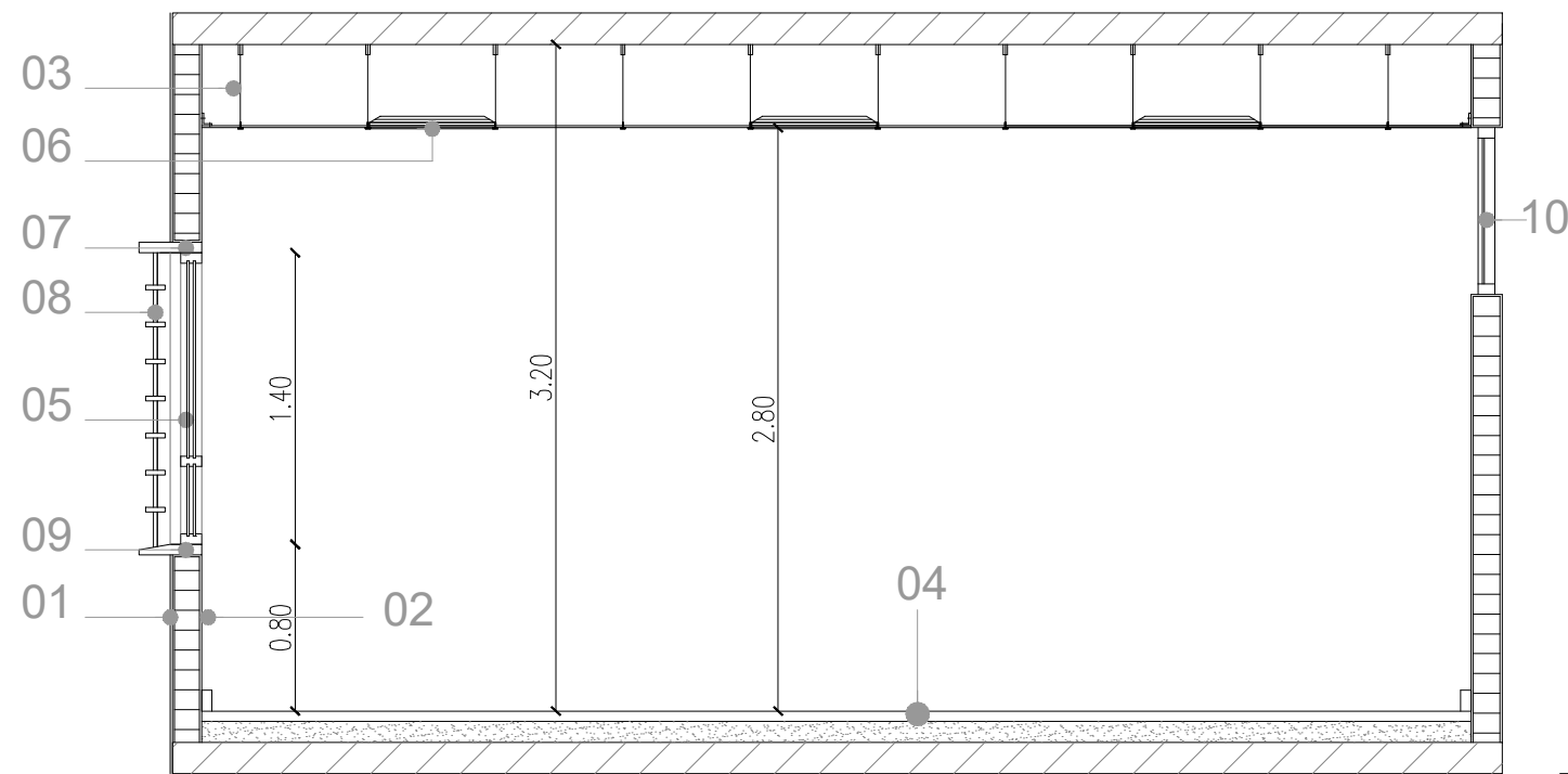
CORTE AULA
