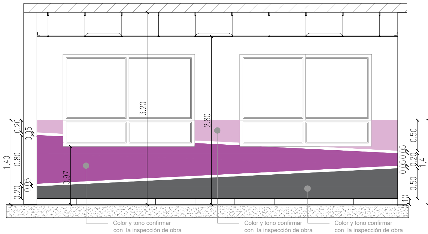
CORTE AULA
