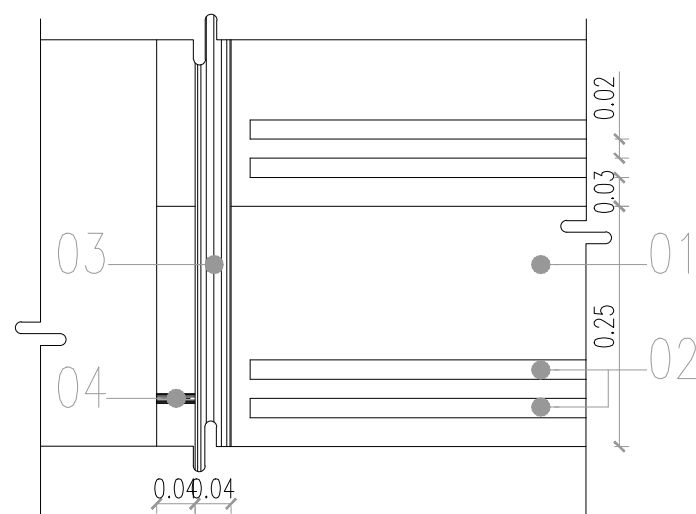
DETALLE 1
