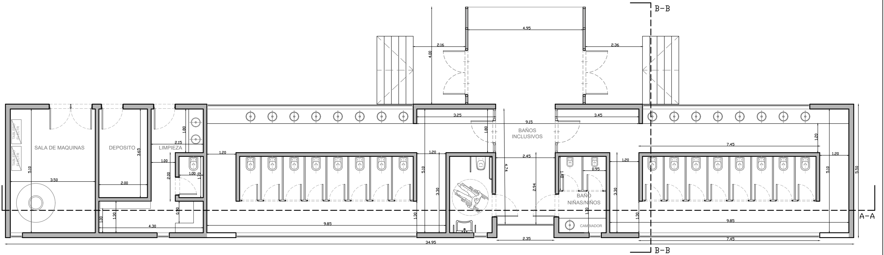
PLANTA BAJA
